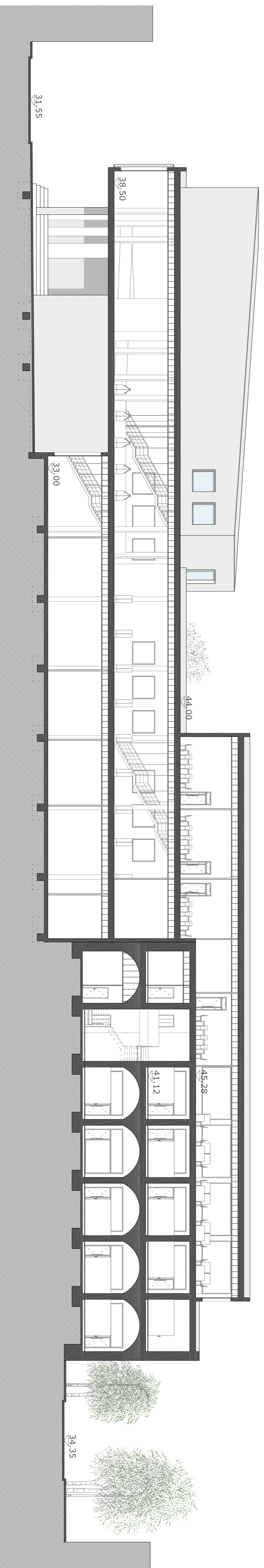
SECCIÓ L-L'
