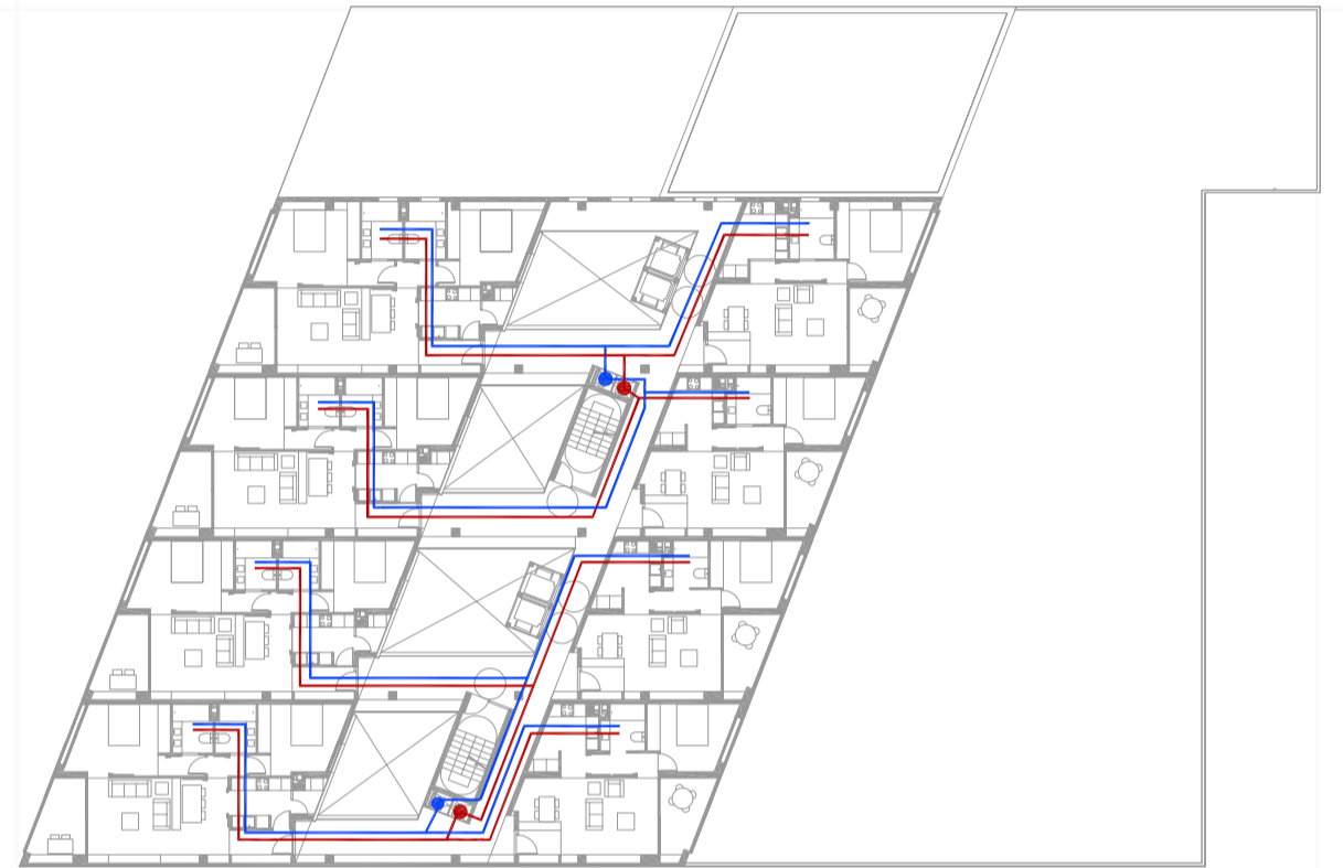
PLANTA TIPUS
