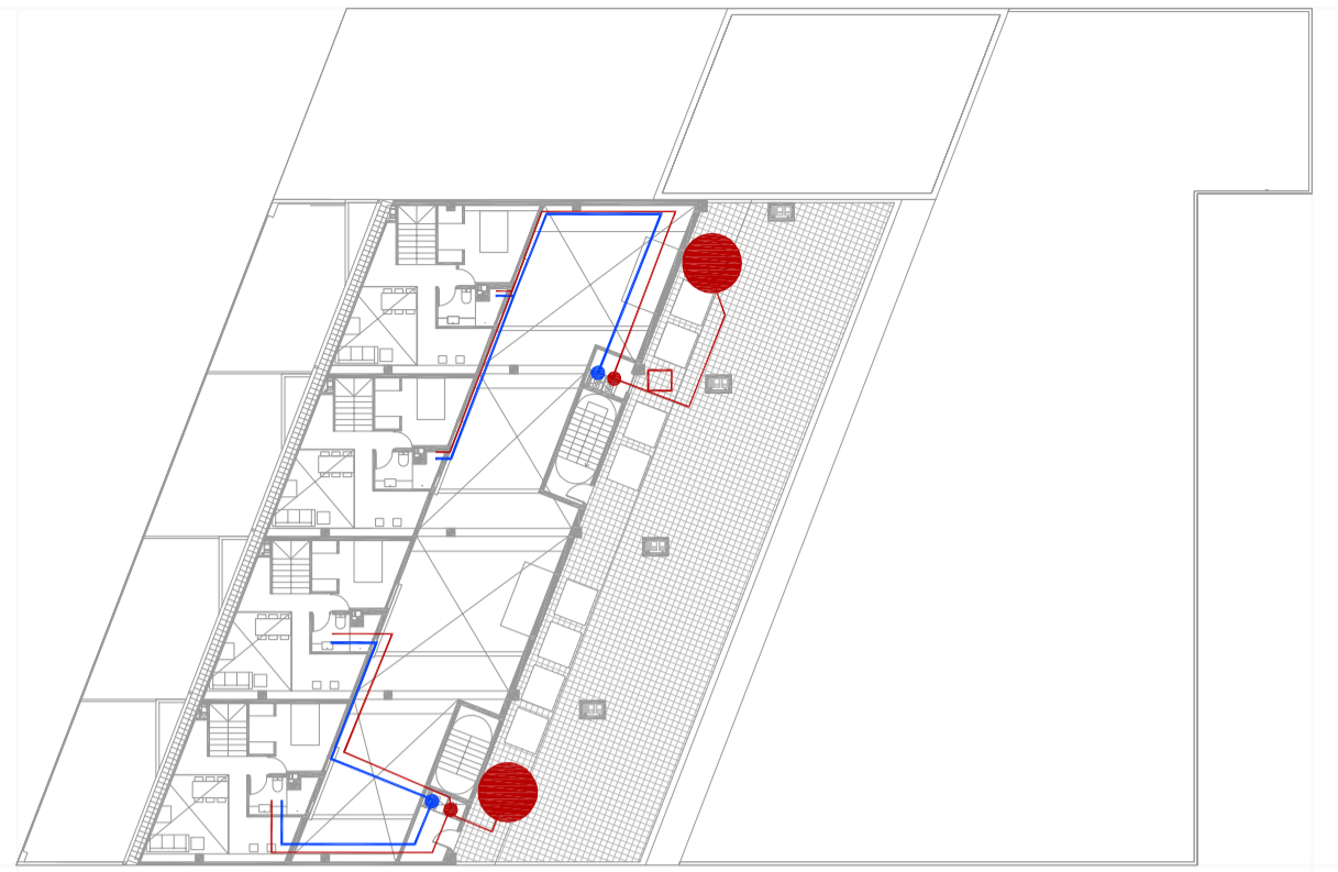
PLANTA SOTACOBERTA
