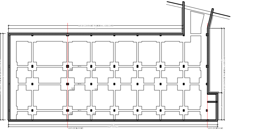
Fonamentació
