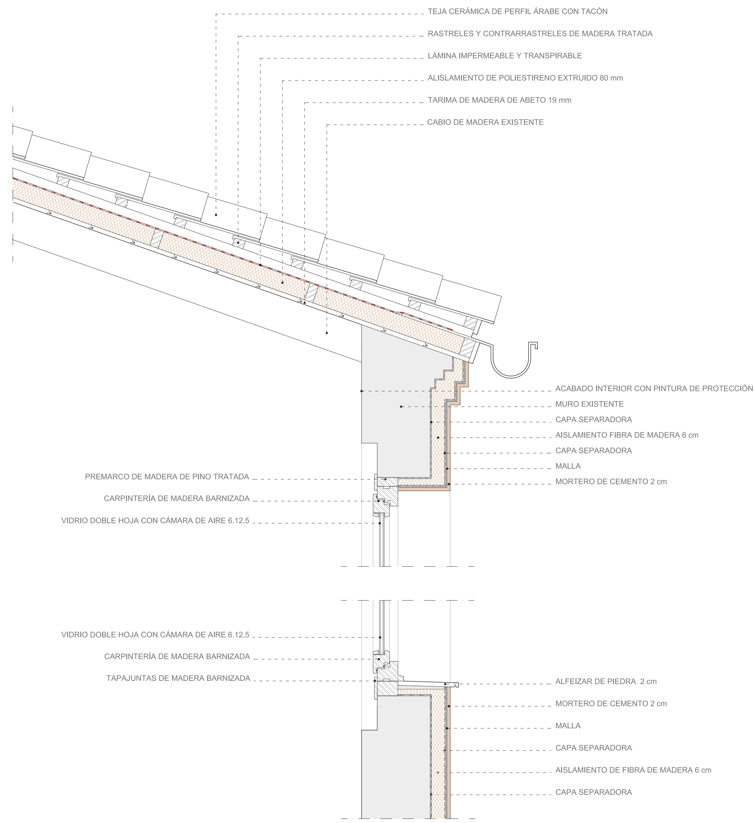
Sección constructiva C E 1:10
