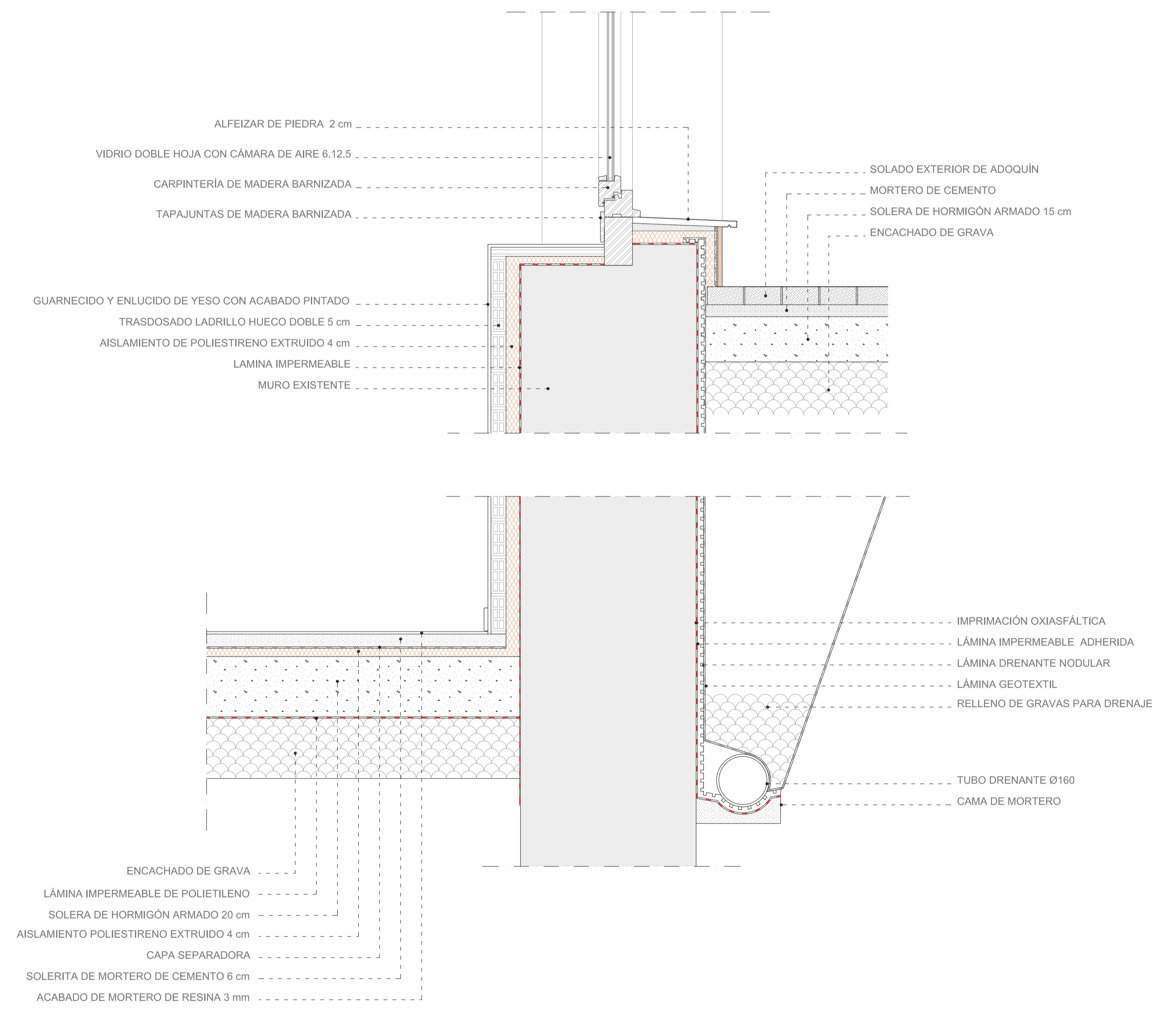
Sección constructiva D E 1:10
