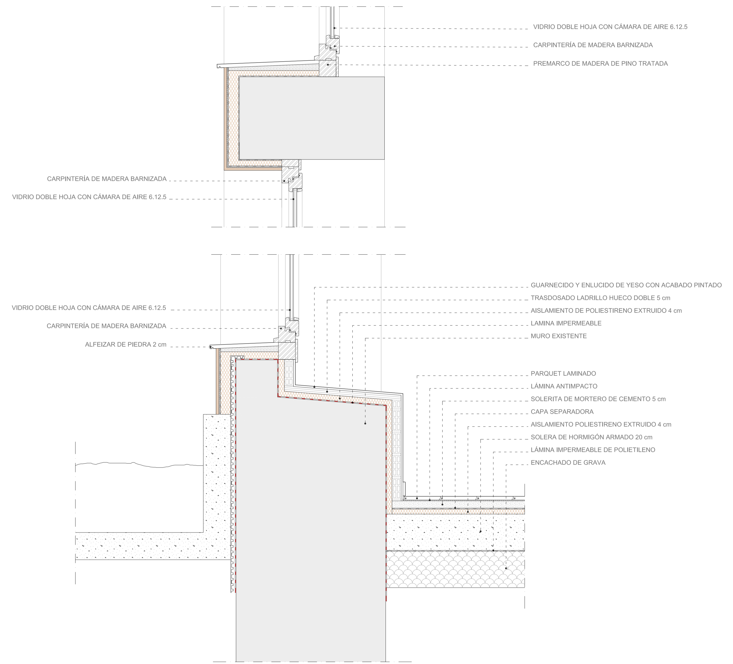
Sección constructiva B E 1:10
