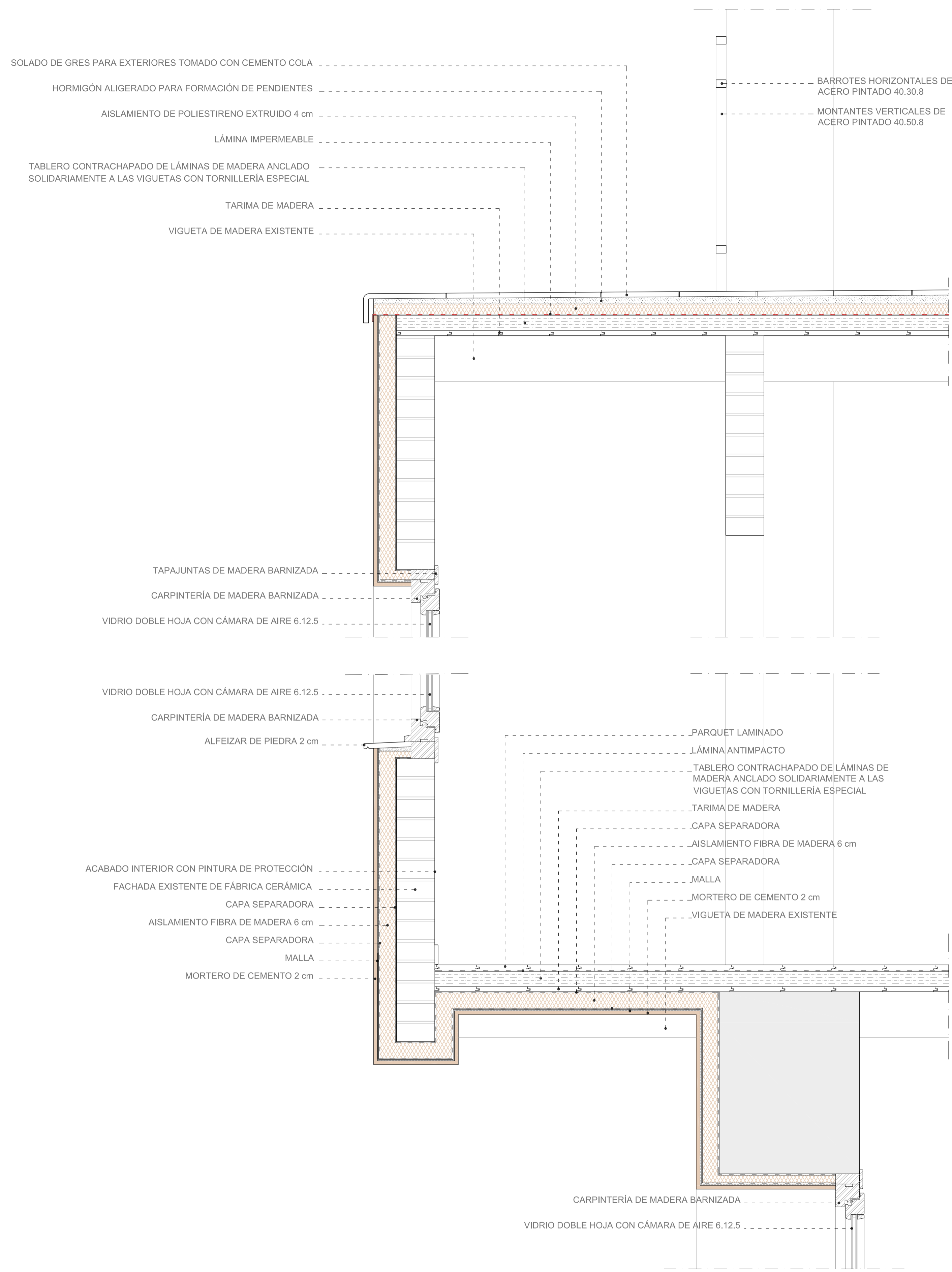
Sección constructiva A E 1:10
