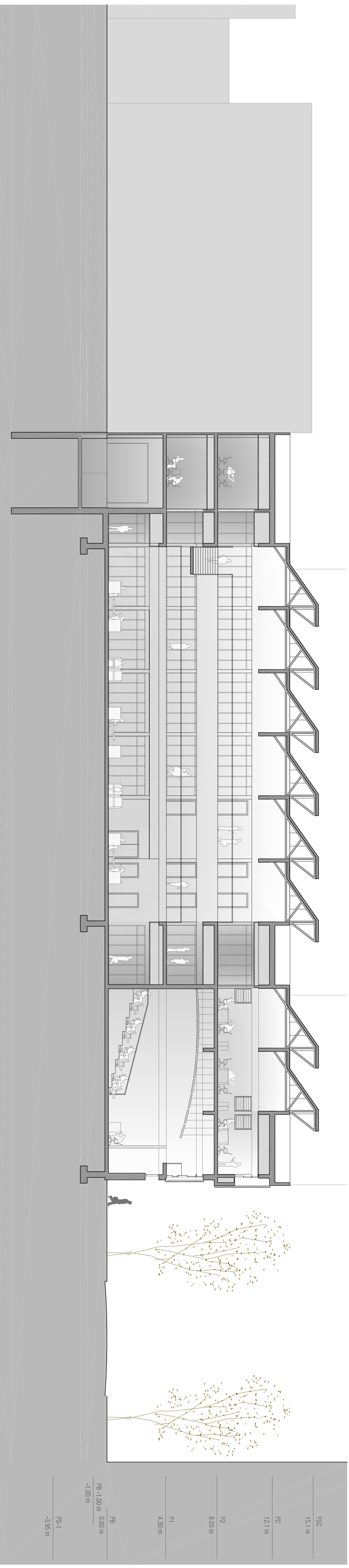
SECCIÓ LONGITUDINAL 2 E. 1/150
