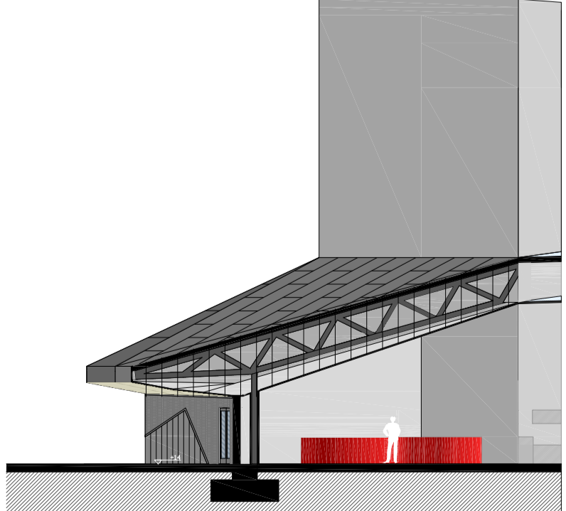
_Secció per l'accés principal, a-a'
