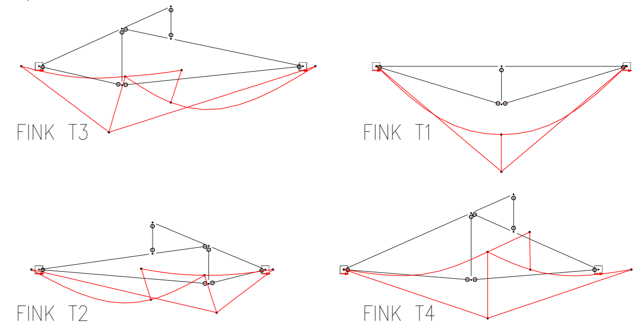
4 - Diagrama de deformació degut a totes les càrregues que haguessim obtingut sense l'efecte del pretensat
