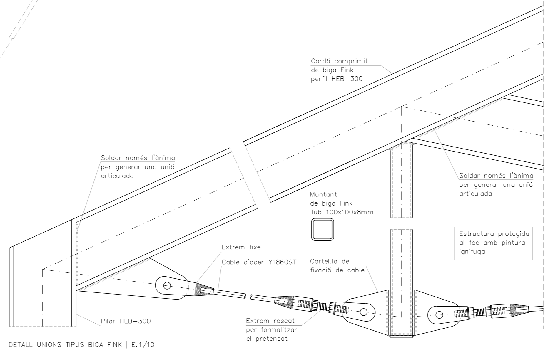
DETALL UNIONS TIPUS BIGA FINK | E:1/10
