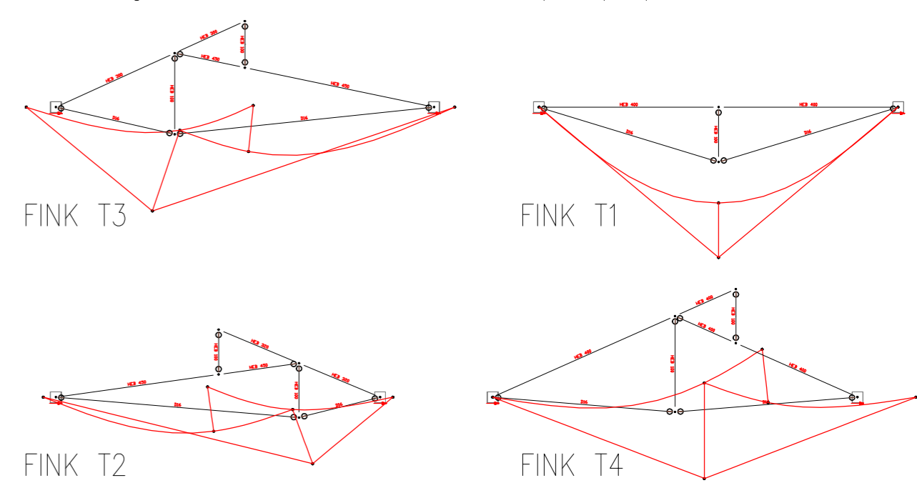
2 - Apliquem una acció de pretensat per tal de compensar la deformació anterior
