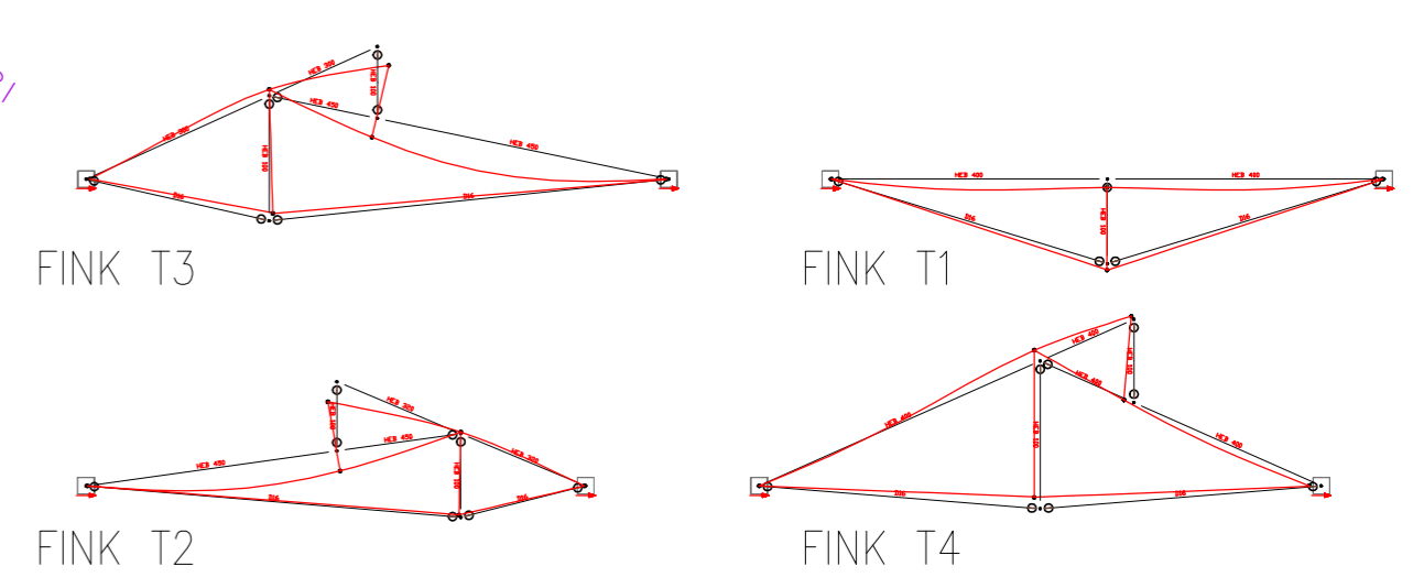
3 - Diagrama de deformació final aplicant la resta de càrregues (permanents i variables) després d'haver pretensat - Cumpnim L/350 de fletxa total
