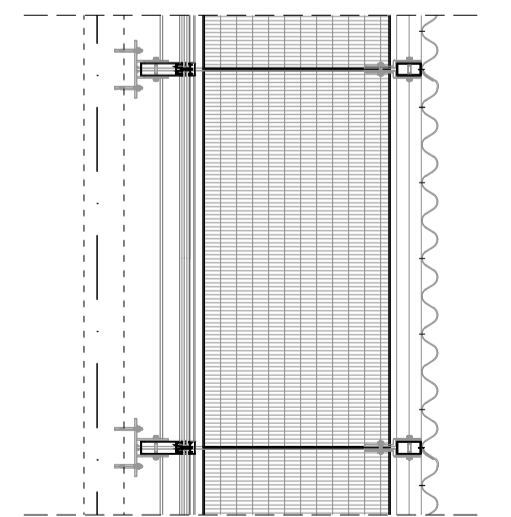
Pell interior: mur cortina vidre Pell exterior: obertura
