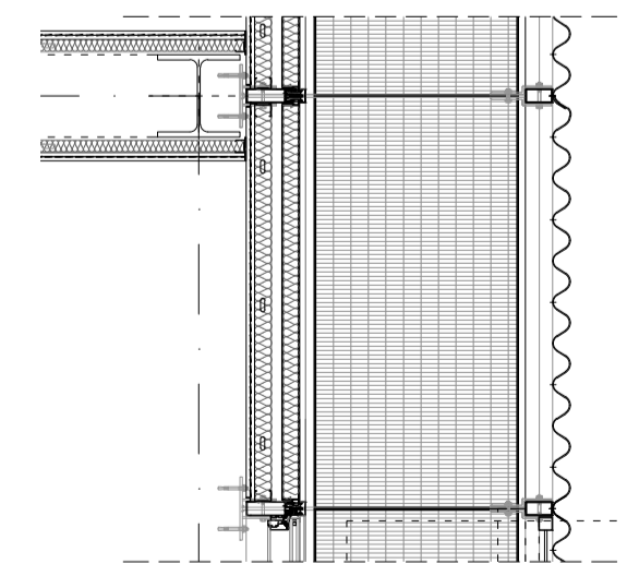
Pell interior: mur cortina panell d'alumini amb aïllant Pell exterior: panell de policarbonat
