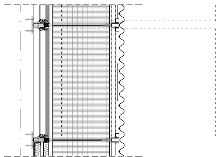
Pell interior: mòdul de finestra practicable Pell exterior: mòdul amb panell practicable motoritzat de policarbonat (tancat)
