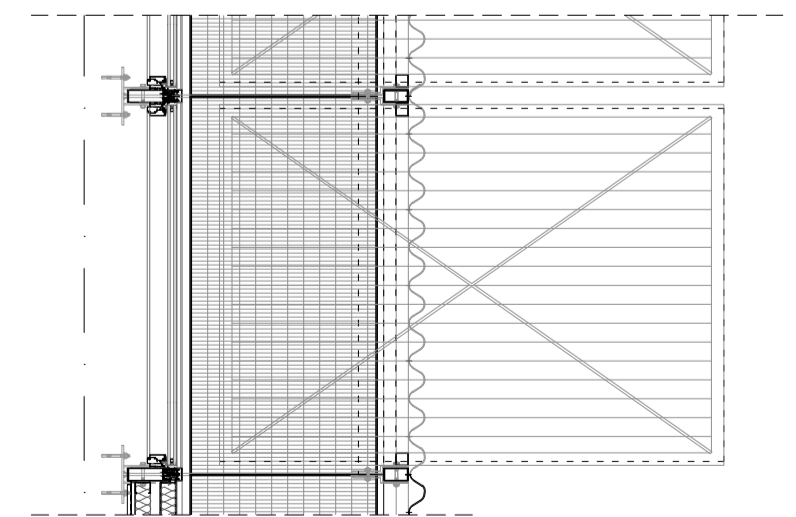
Pell interior: mòdul de finestra practicable Pell exterior: mòdul amb panell practicable motoritzat de policarbonat (obert)
