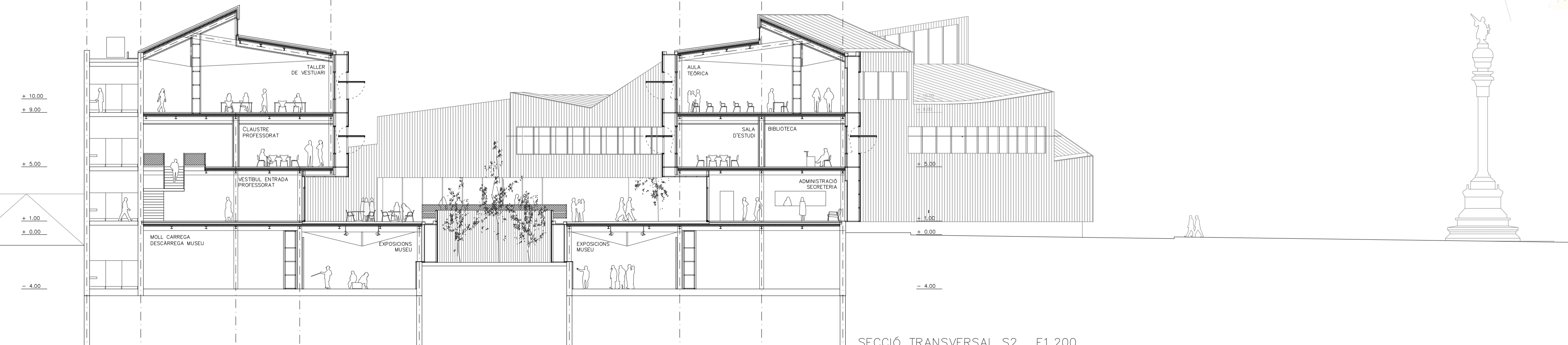
SECCIÓ TRANSVERSAL S2 . E1.200
