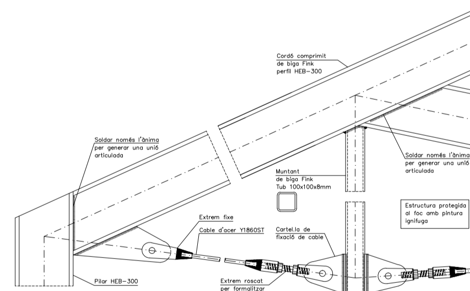
DETTALL UNIONS TIPUS BIGA FINK . E1.10
