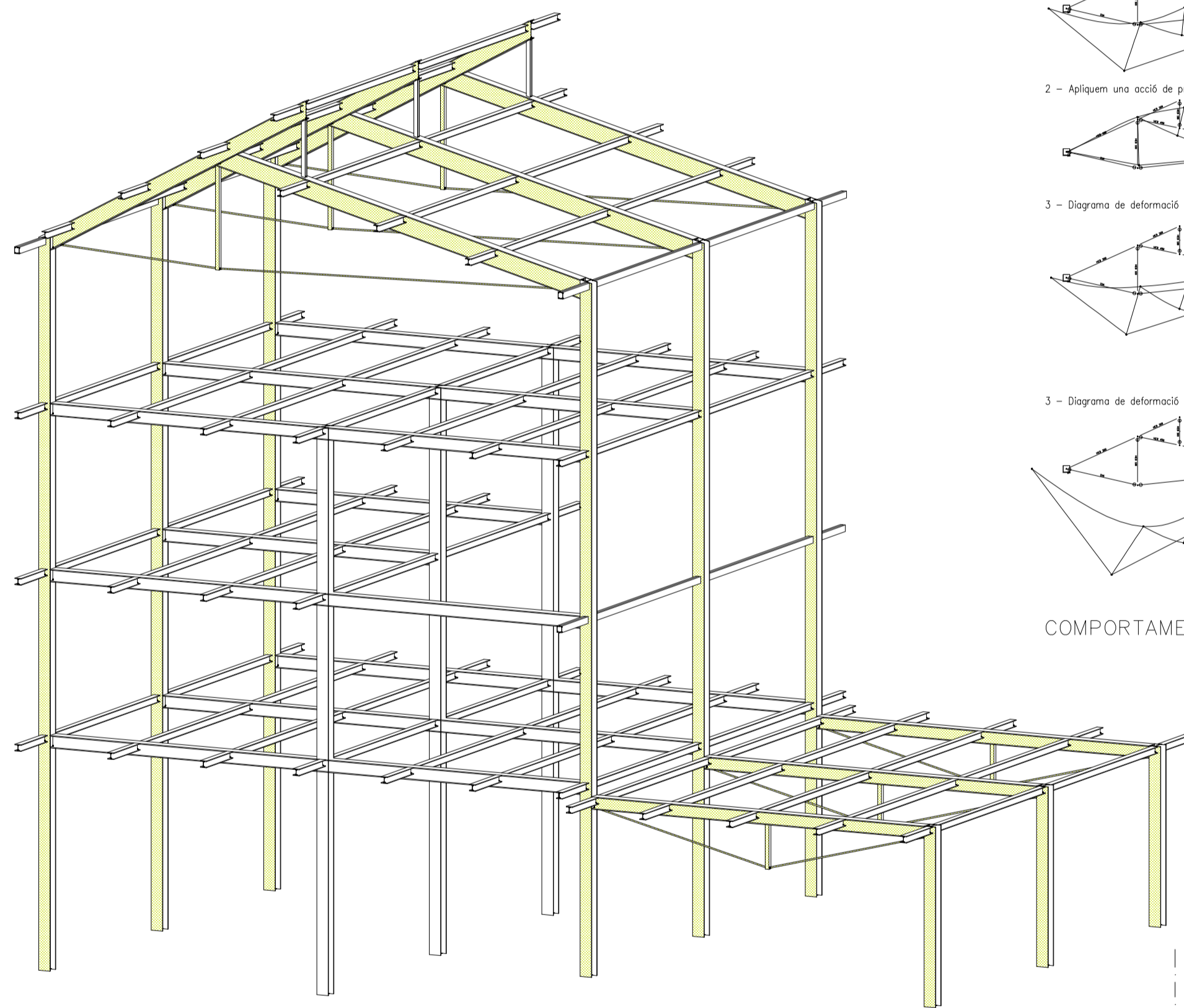
ESQUEMA ESTRUCTURAL
