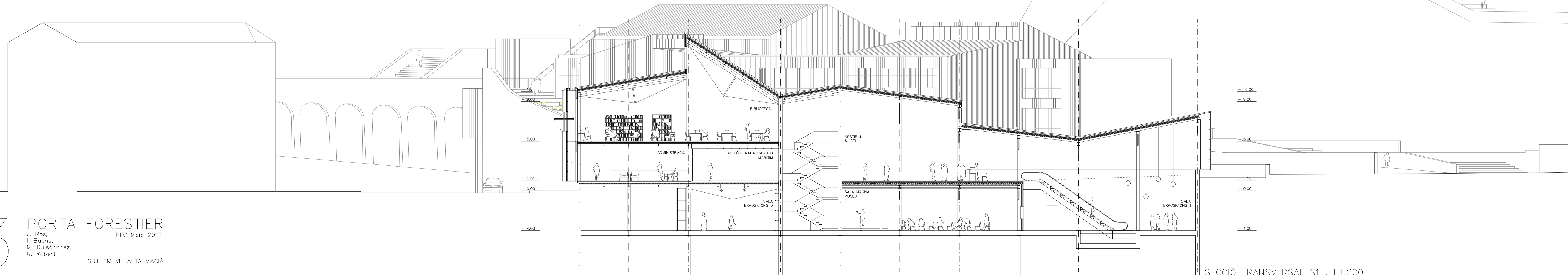
SECCIÓ TRANSVERSAL S1 . E1.200
