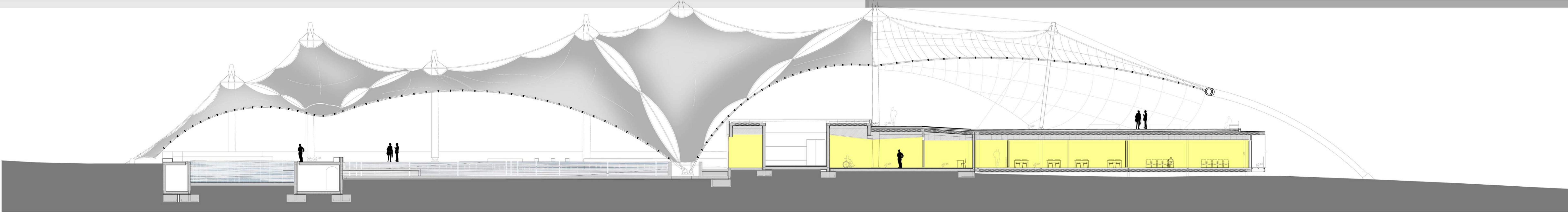
SECCIÓ C-C'_1:150
