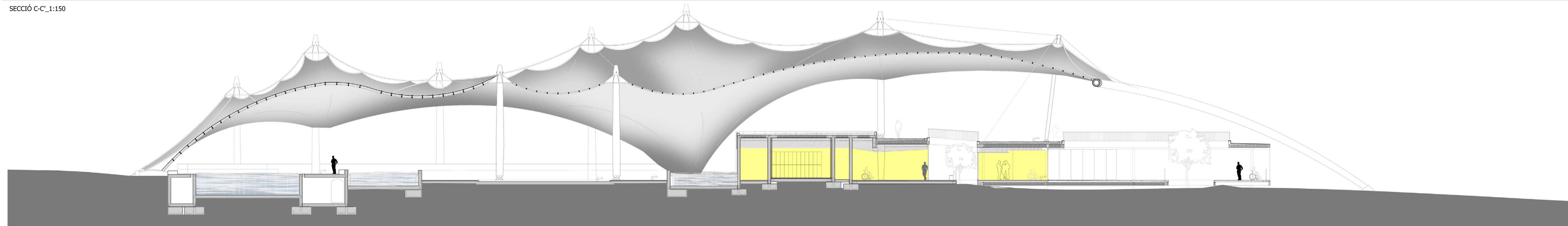
SECCIÓ D-D'_1:150
