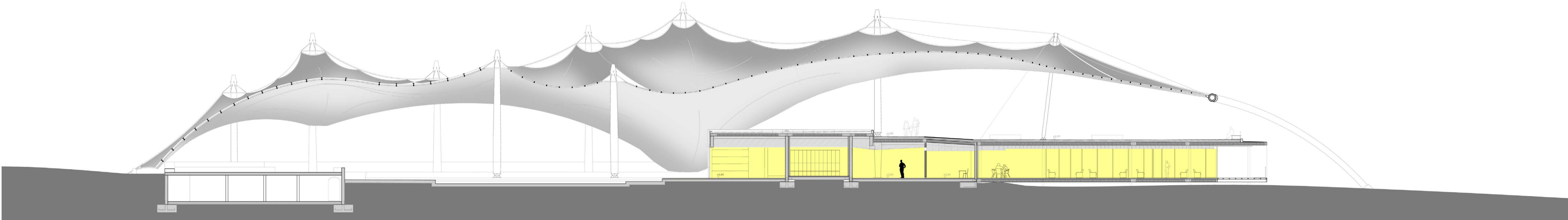
SECCIÓ E-E'_1:150
