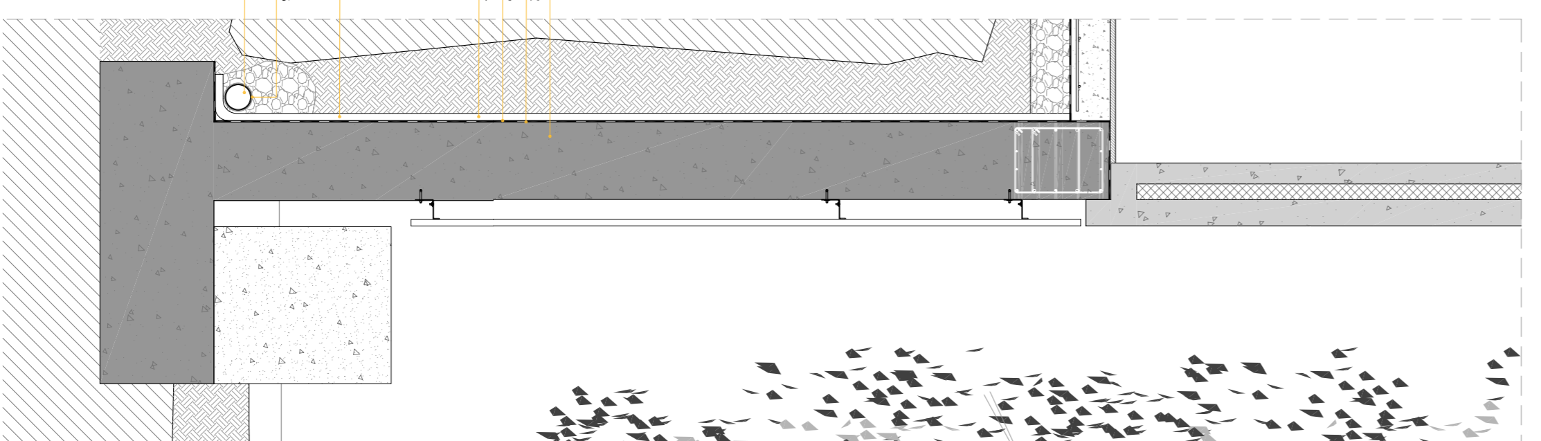
SECCIÓ DETAL CONSTRUCTIU BIBLIOTECA DE BARRI 1/20
