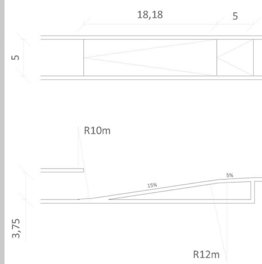
PLANTA I SECCIÓ RAMPA D'ACCÉS 1/300
