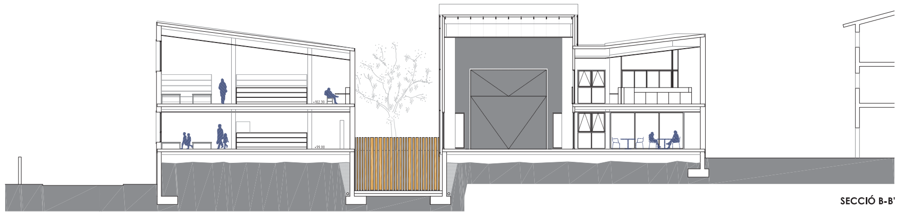
SECCIÓ A-A'
