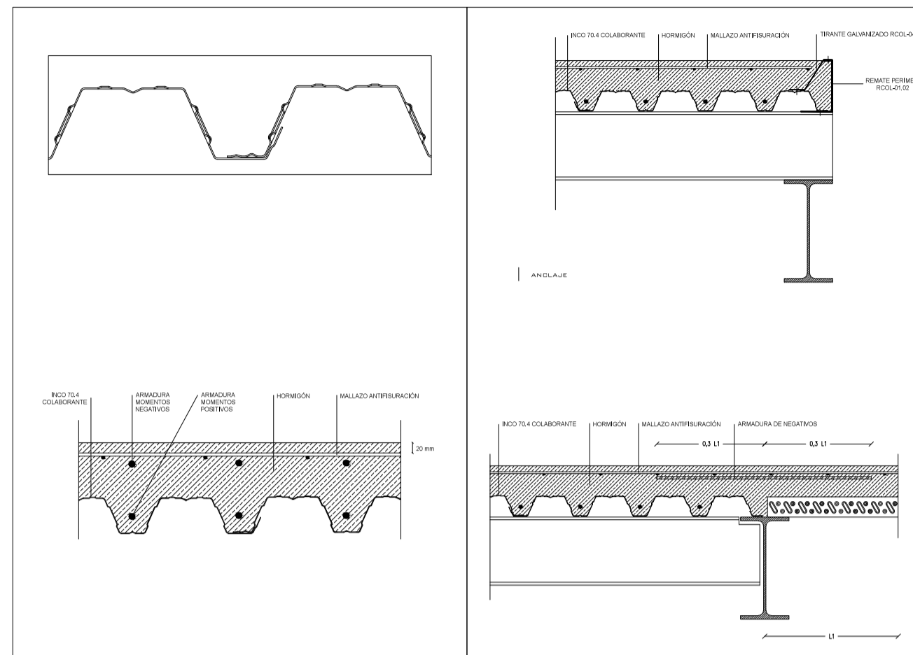
ESQUEMES I DETALLS FORJAT COLABORANT E:1/75
