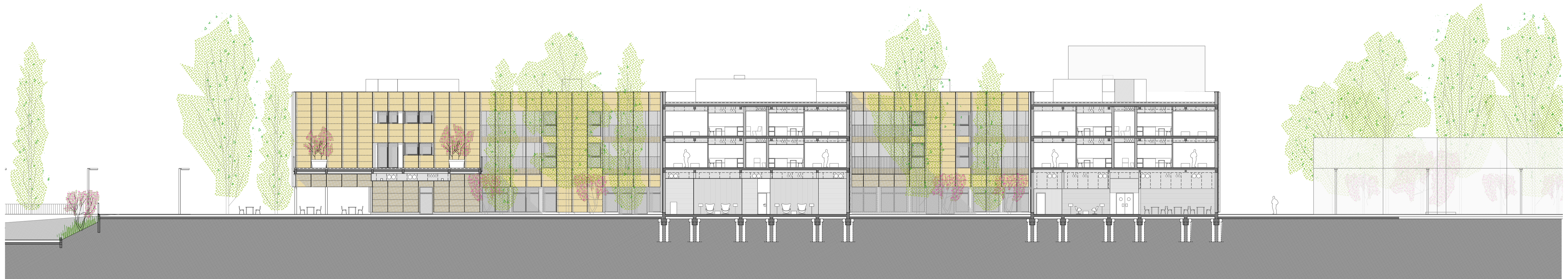
SECCIÓ LONGITUDINAL SL 02
