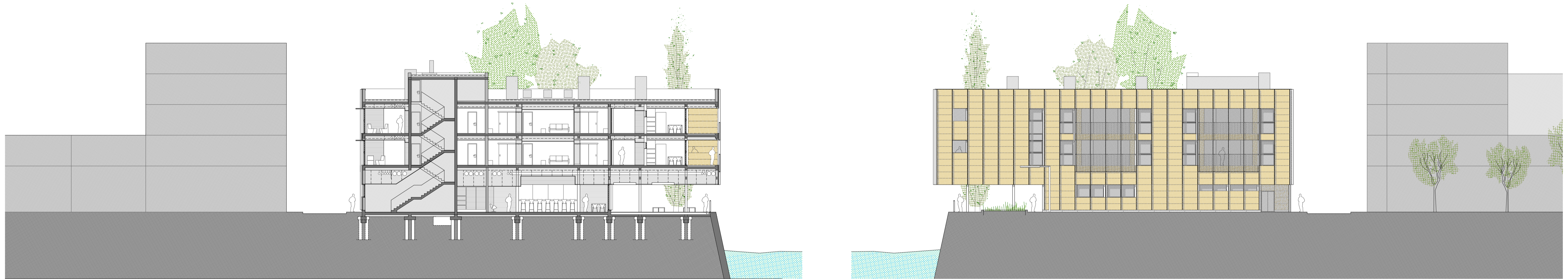
ALÇAT PLAÇA DE L'AUBE
