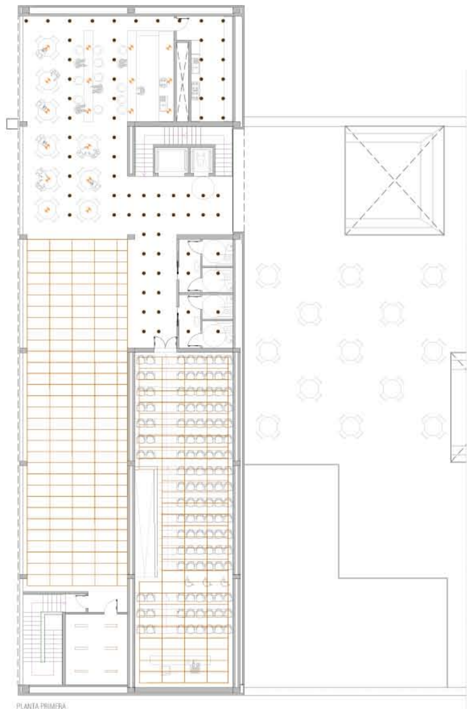
PLANTA PRIMERA
