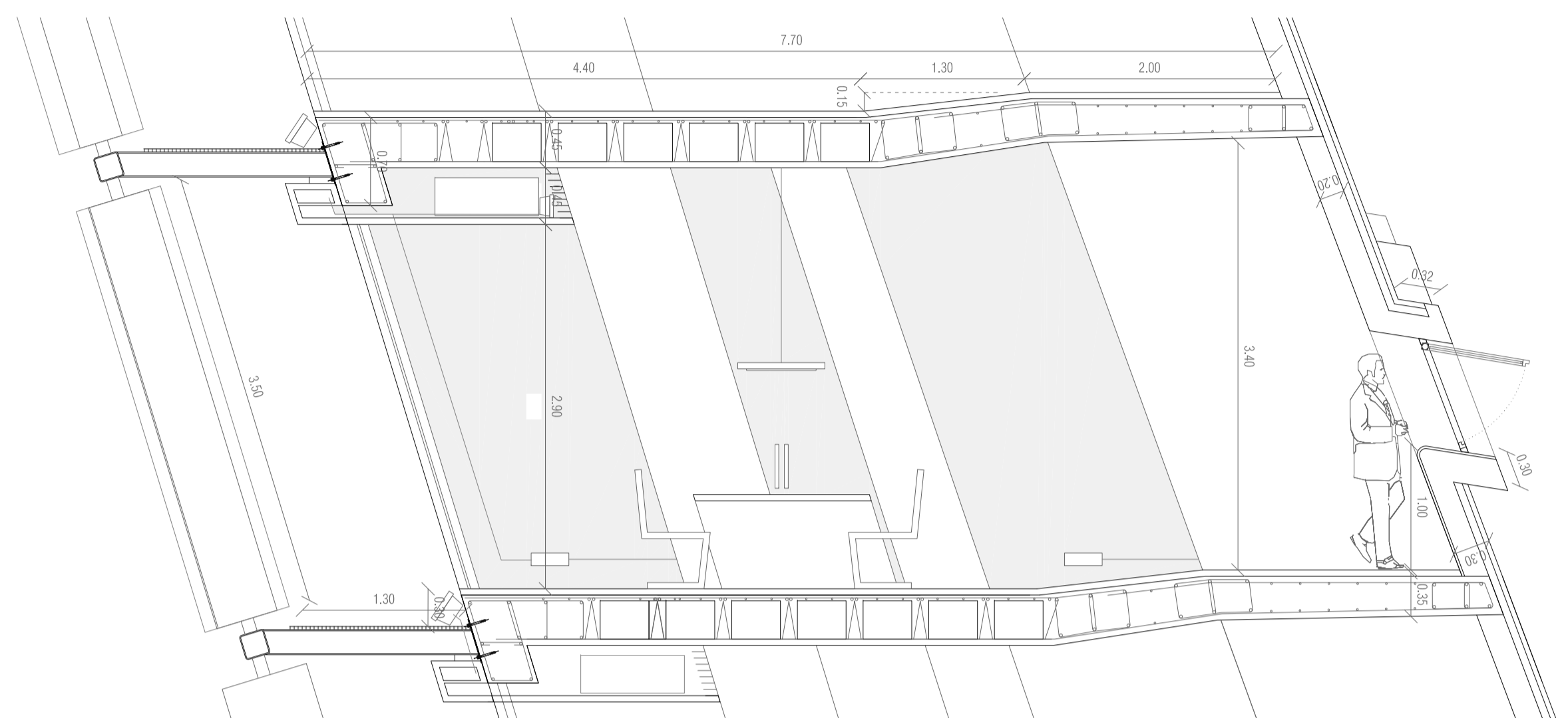
SECCIÓ OFICINA TIPUS E. 1/40
