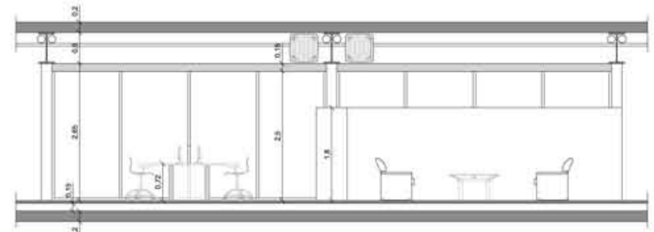
SECCIÓ ESCALA 1:100
