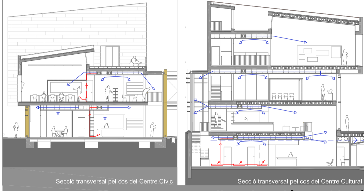
Secció transversal pel cos del Centre Cívic / Secció transversal pel cos del Centre Cultural
