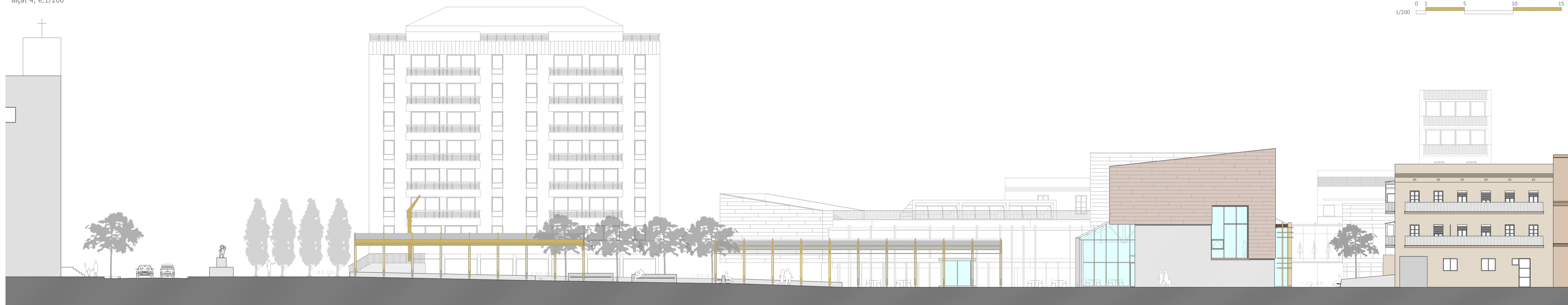
alçat 5, e.1/200
