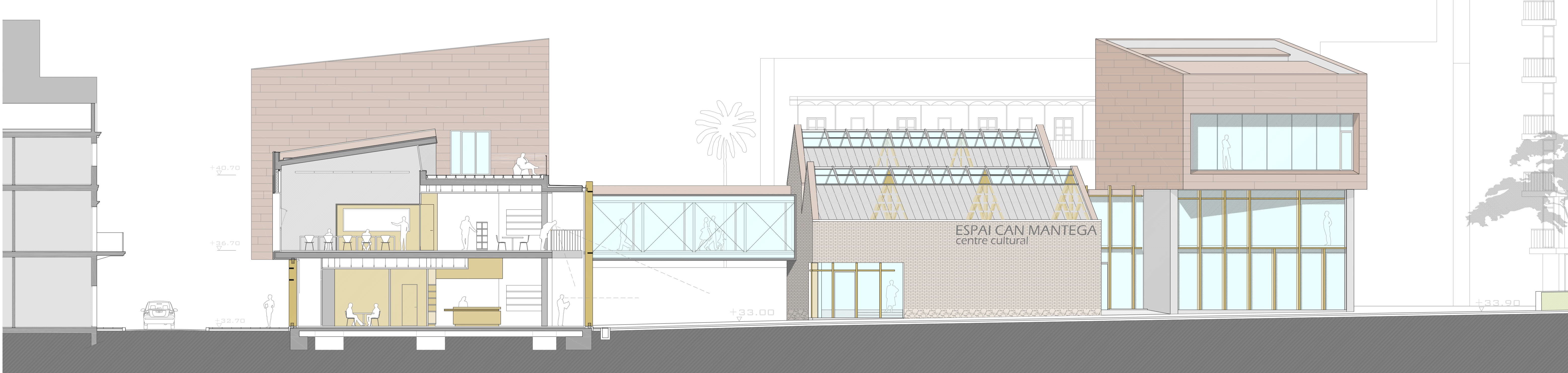
secció 2, e.1/100
