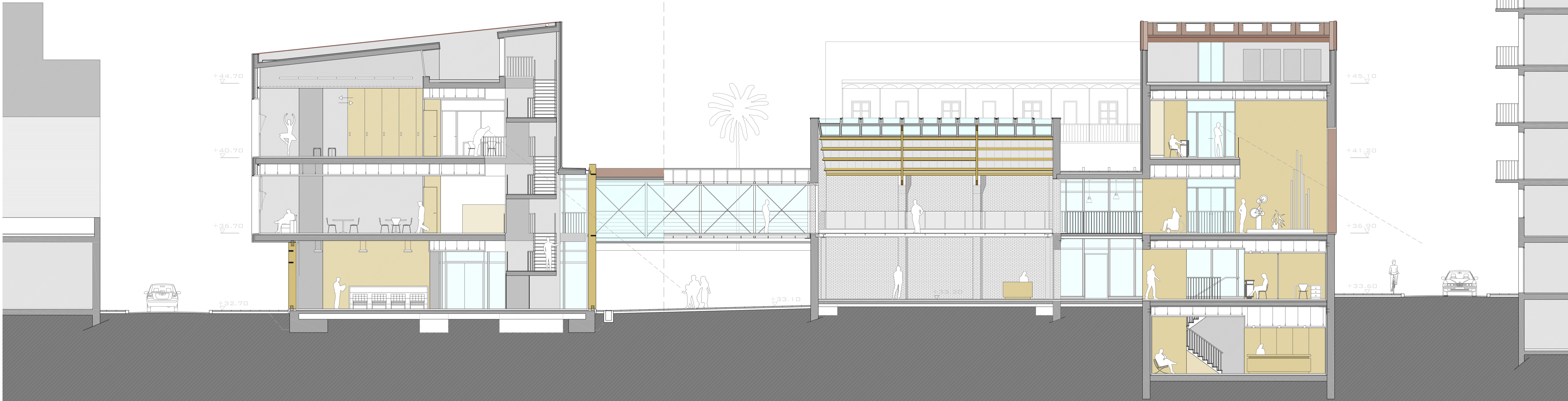
secció 1, e.1/100
