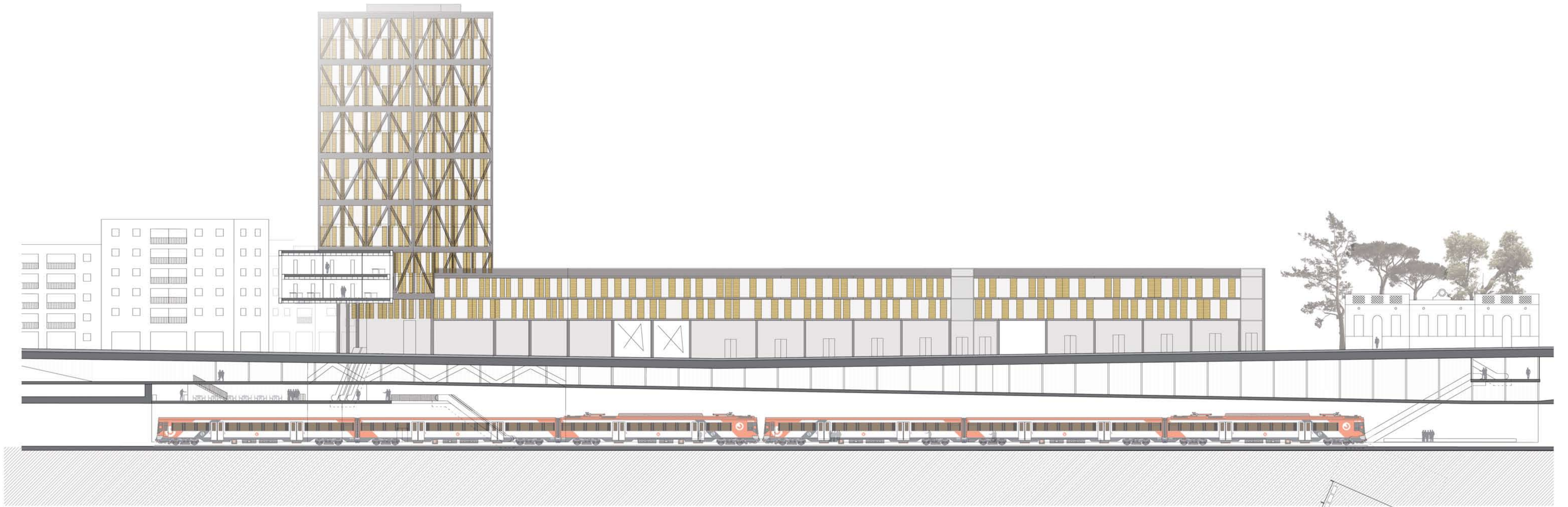
Secció Longitudinal a Sud [e 1/300]
