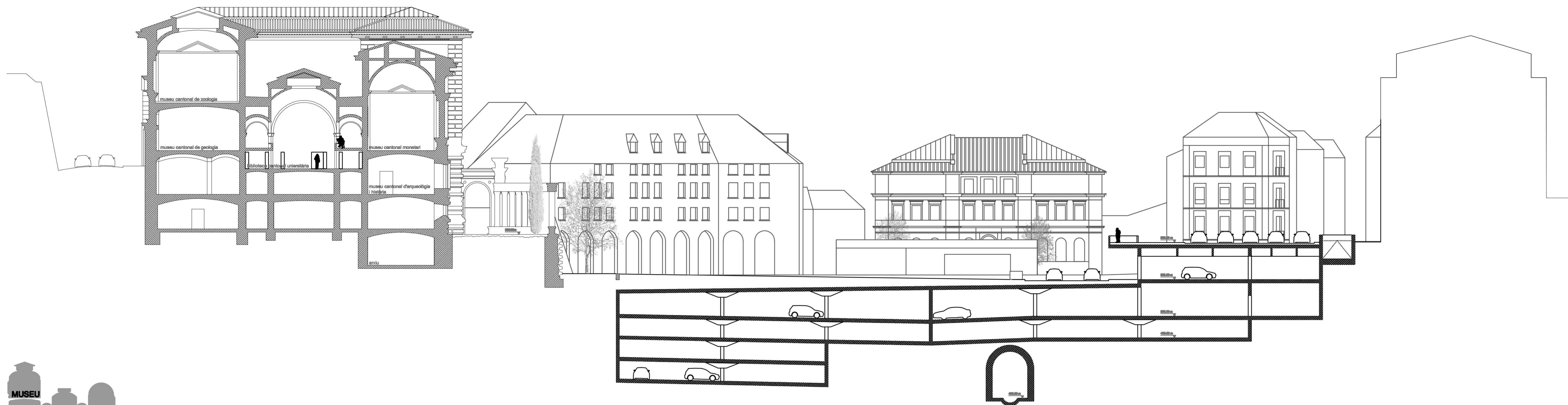
secció transversal per antic cinema romandí estat actual 1/250
