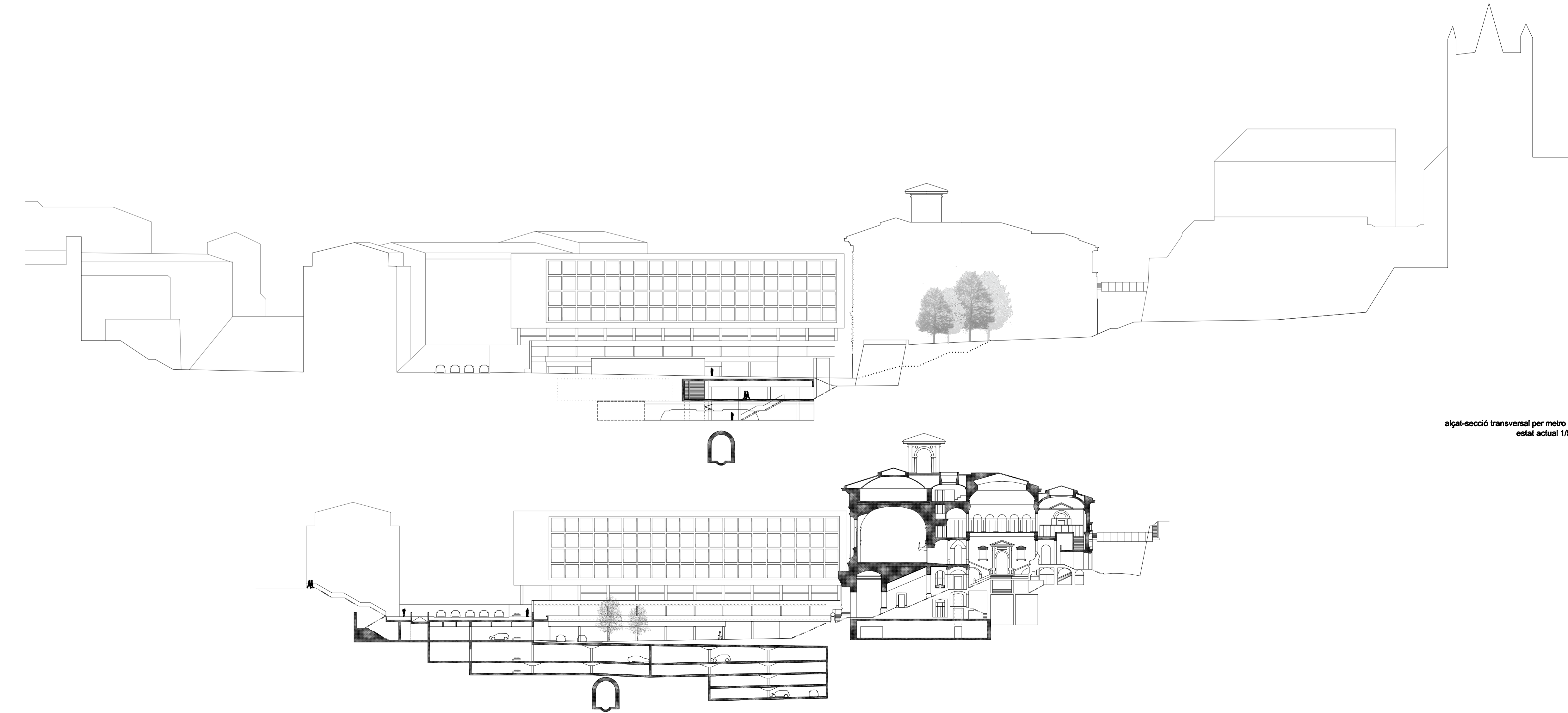
secció transversal per eix del palau de rumino estat actual 1/500
