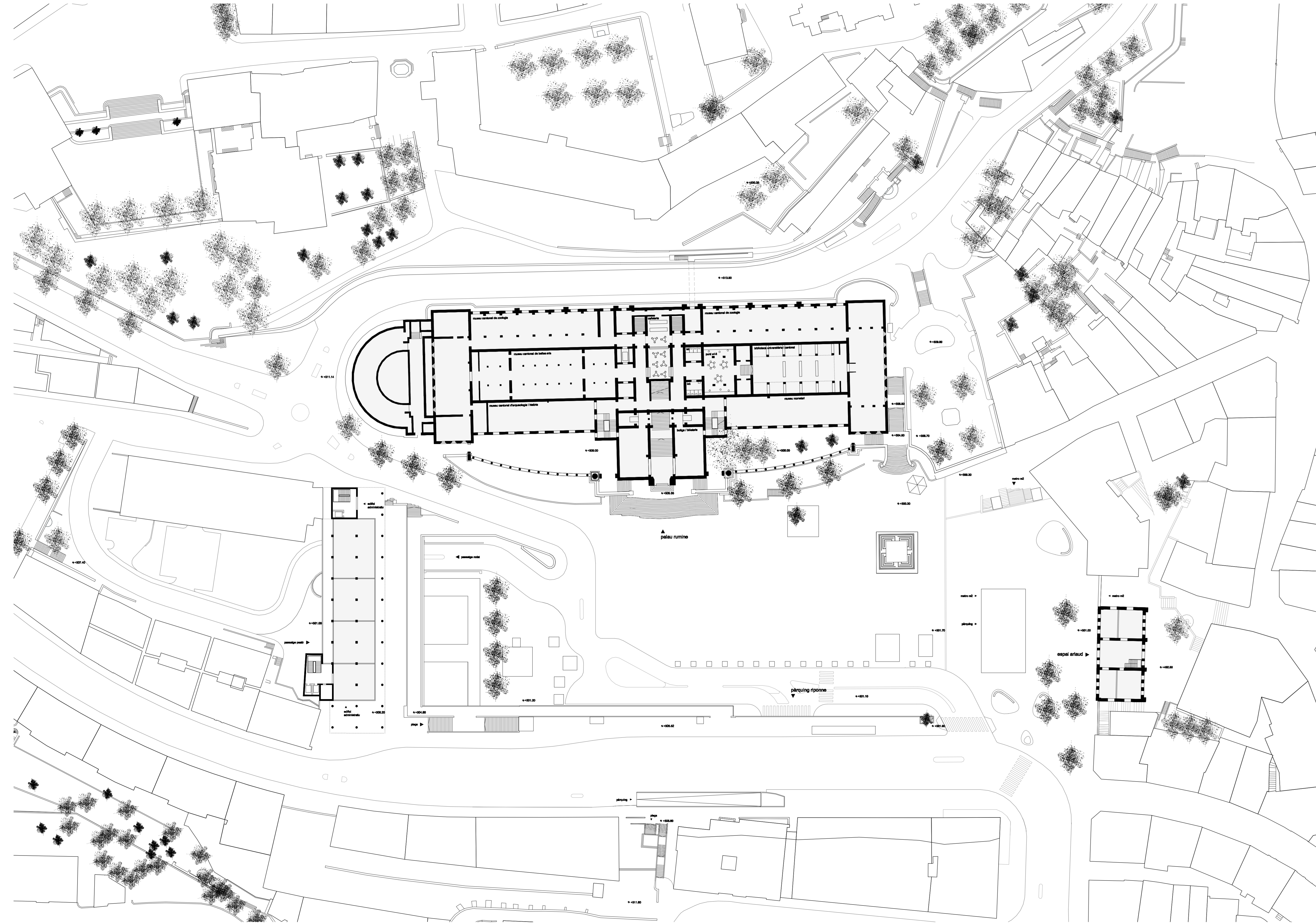
planta plaça riponne estat actual 1/500
