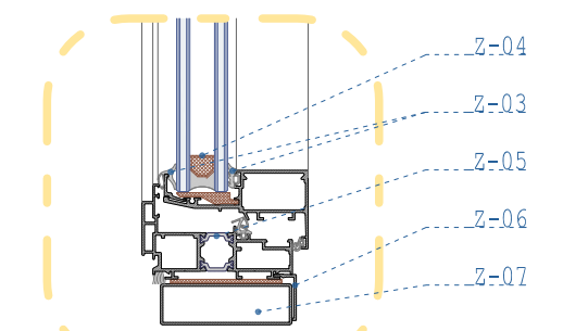
secció vertical, part practicable
