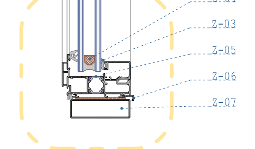
secció vertical, part fixe
