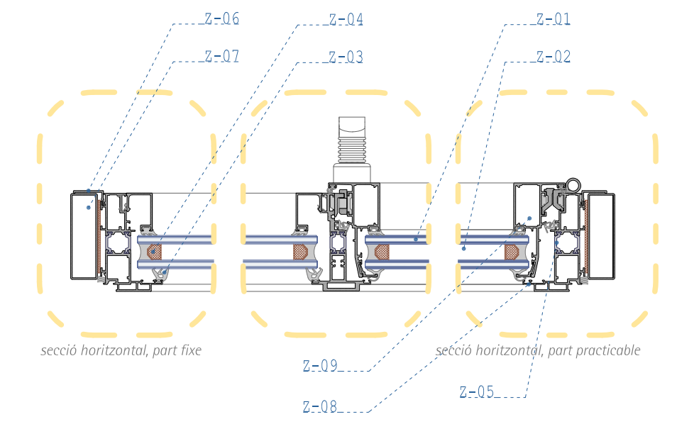
Les fusteries, detalls e: 1/5
