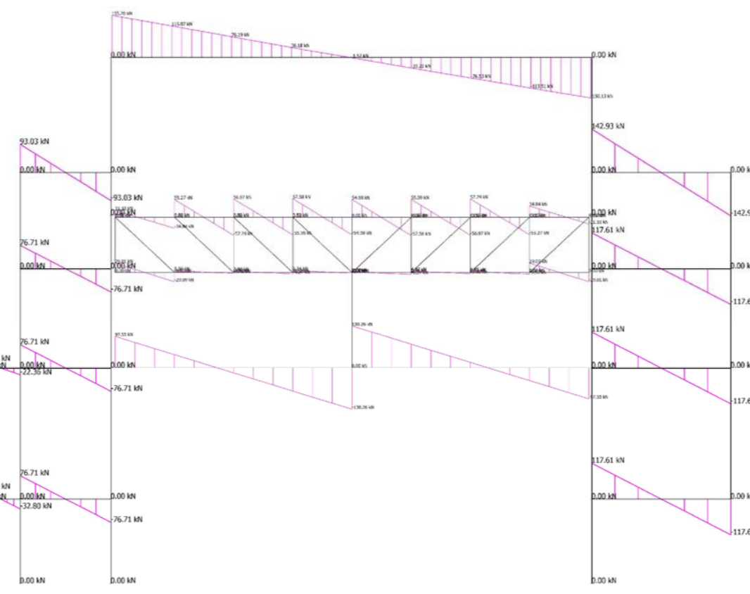
Diagrama de tallans en ELS total
