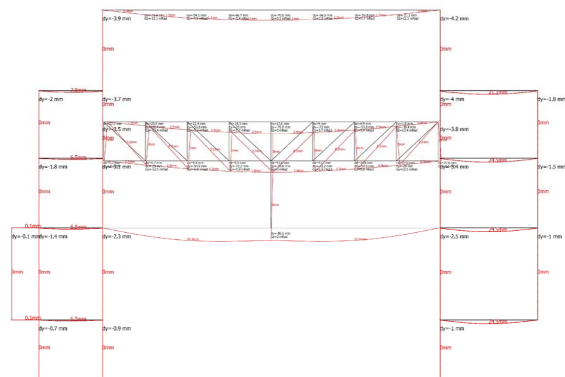
Diagrama de la deformada en ELS total
