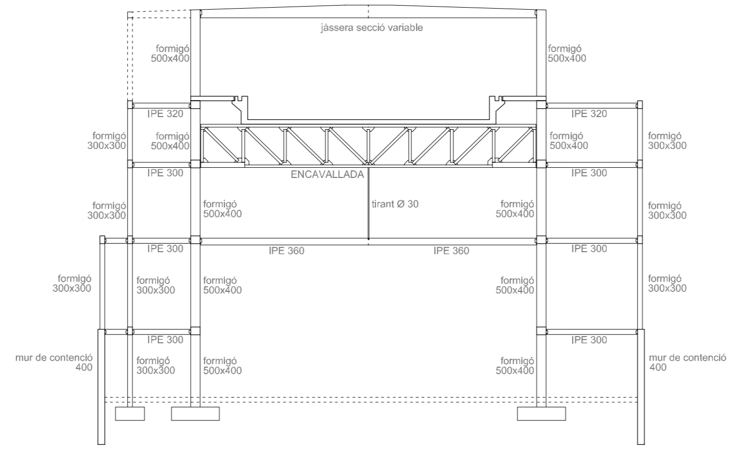
Dimensió del elements portants
