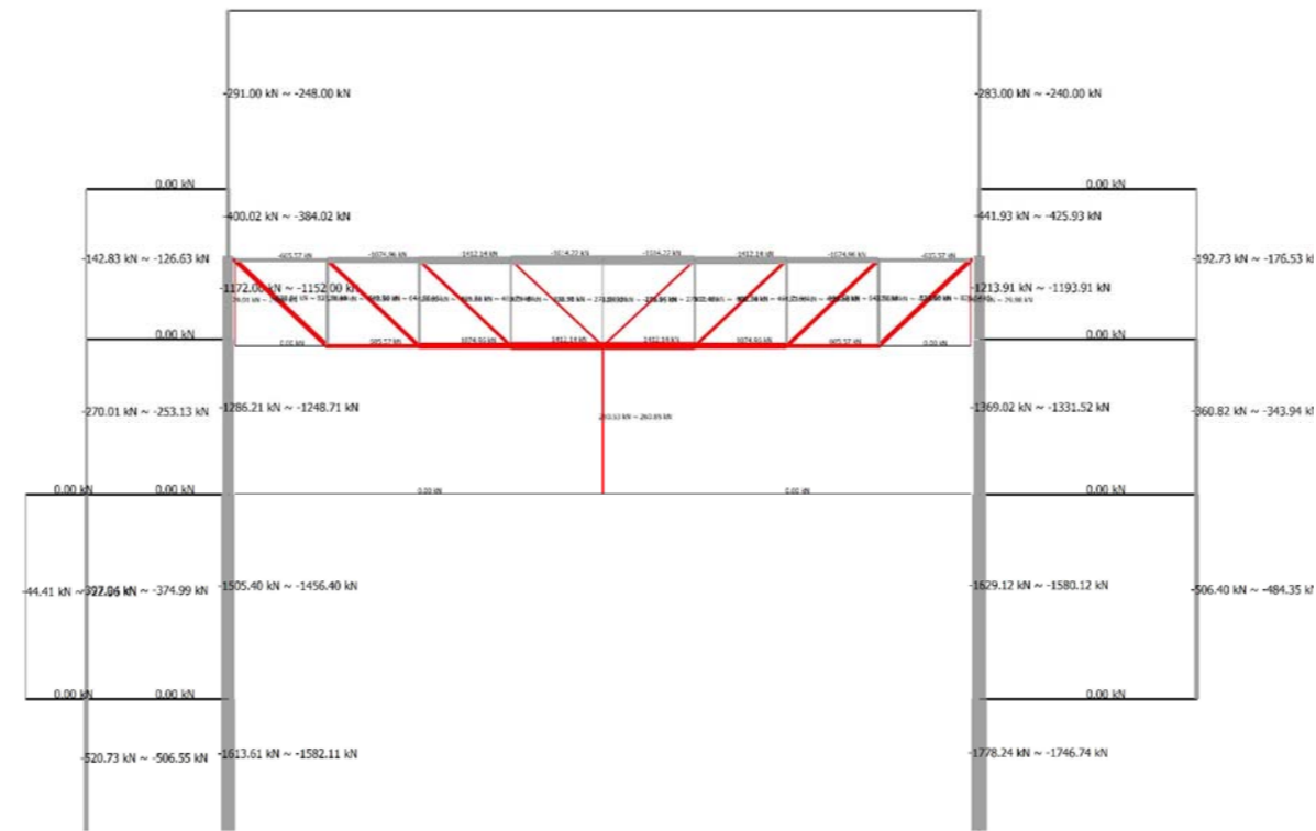
Diagrama de forces axils en ELS total
