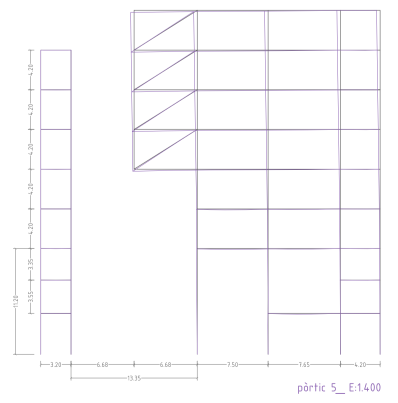
_esquemes deformacions als altres pòrtics principals
