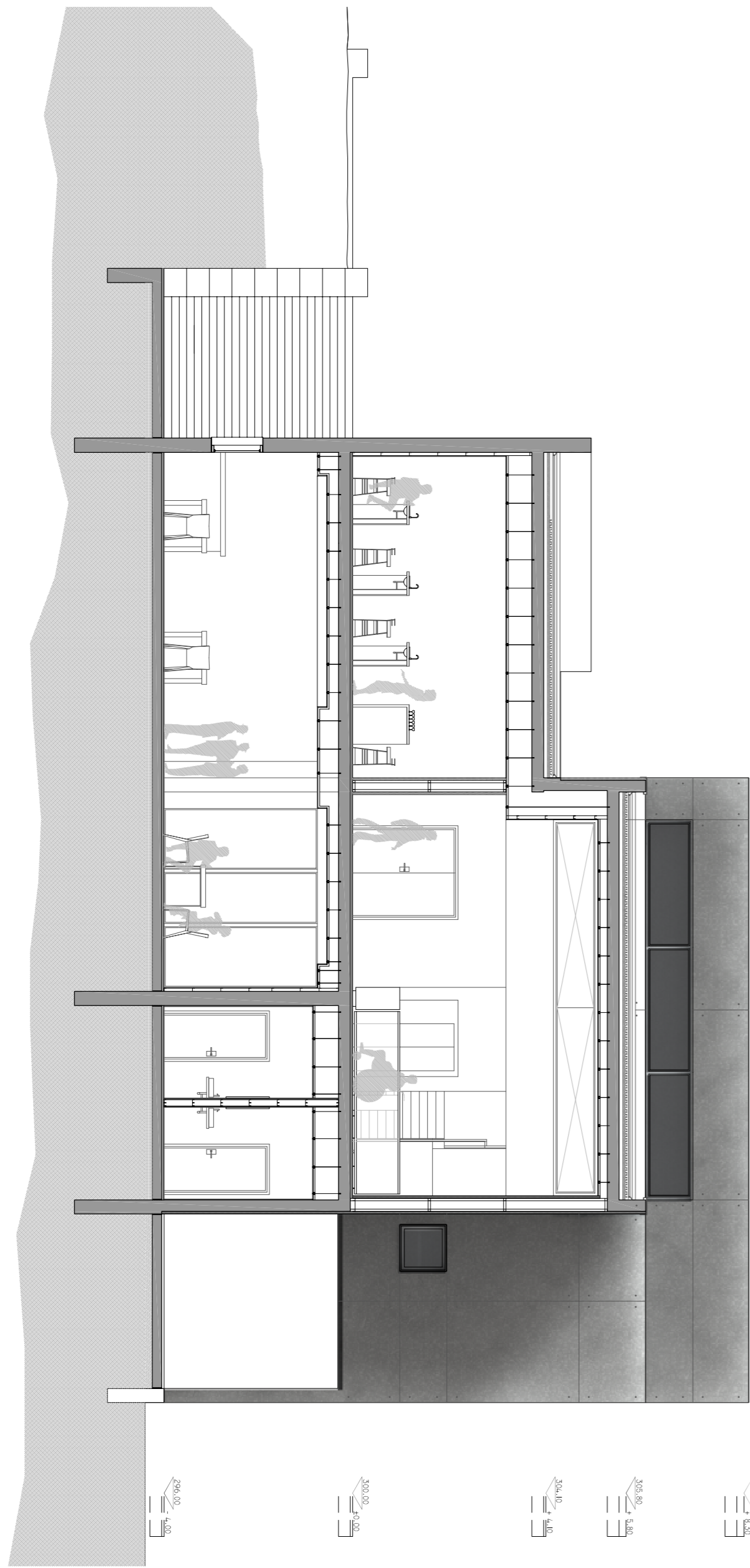
SECCIÓ LONGITUDINAL I-I'
