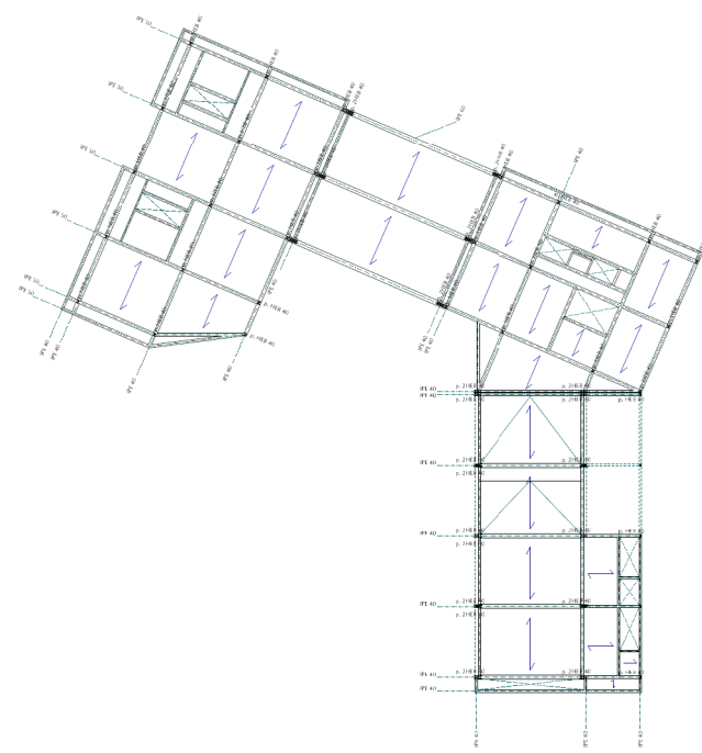
planta altillos 4
