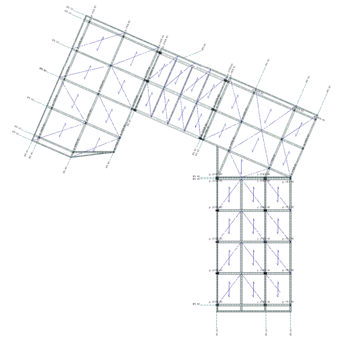
planta cubiertas
