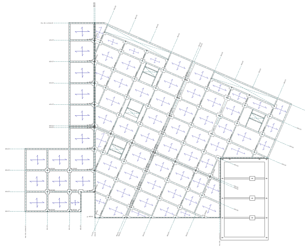
planta aparcamiento 1
