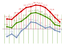
Temperatura media mensual durante el año 2009 (°C)
