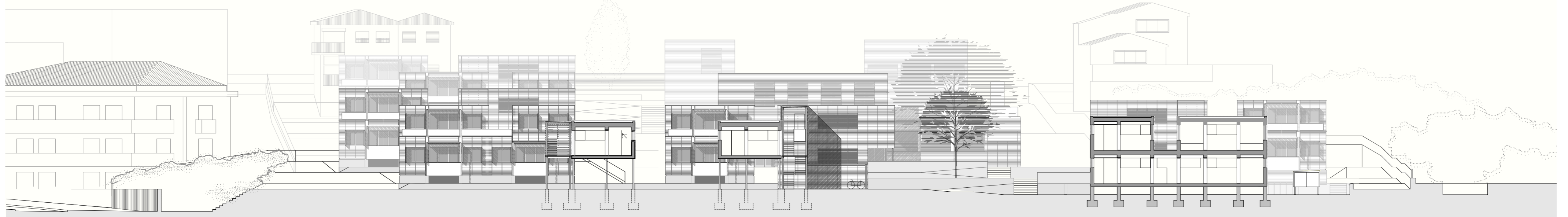
ST01. SECCIÓ TRANSVERSAL PER L'ACCÉS SECUNDARI
