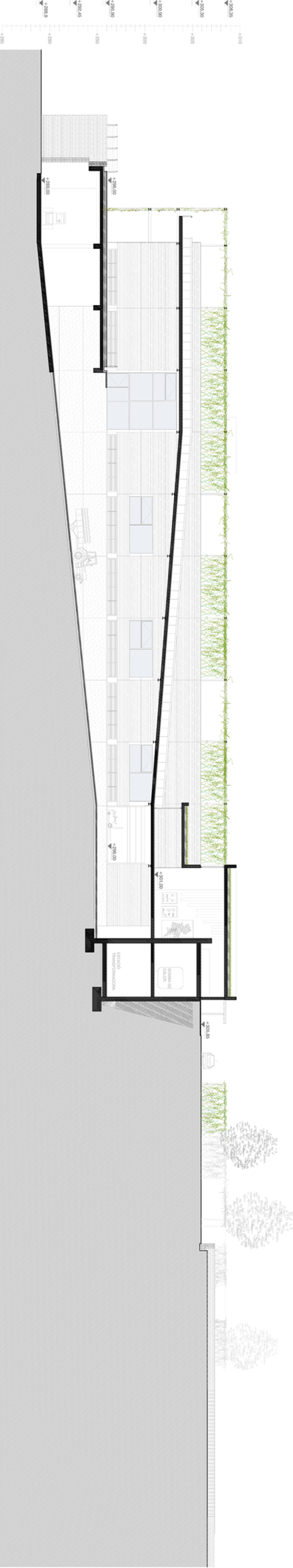
SECCIO LONGITUDINAL 6-6
