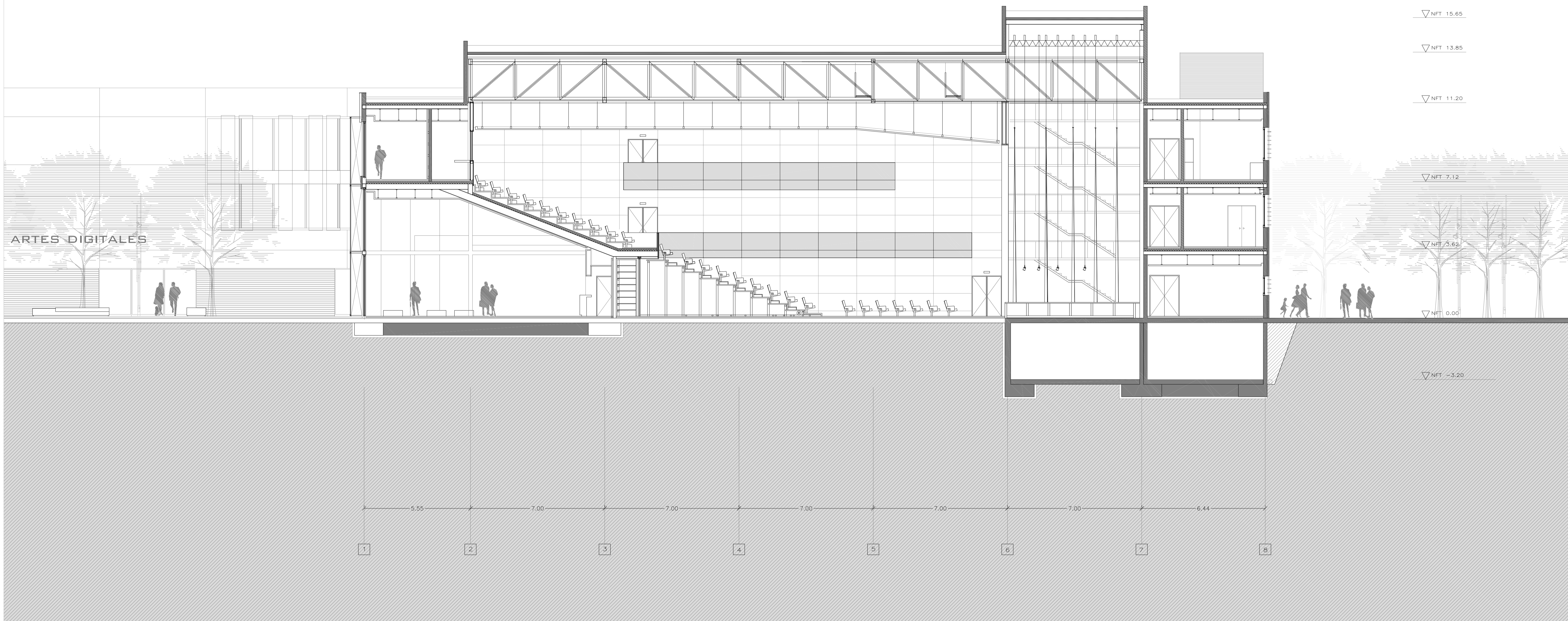
SECCIÓN LONGITUDINAL C-C esc. 1/100
