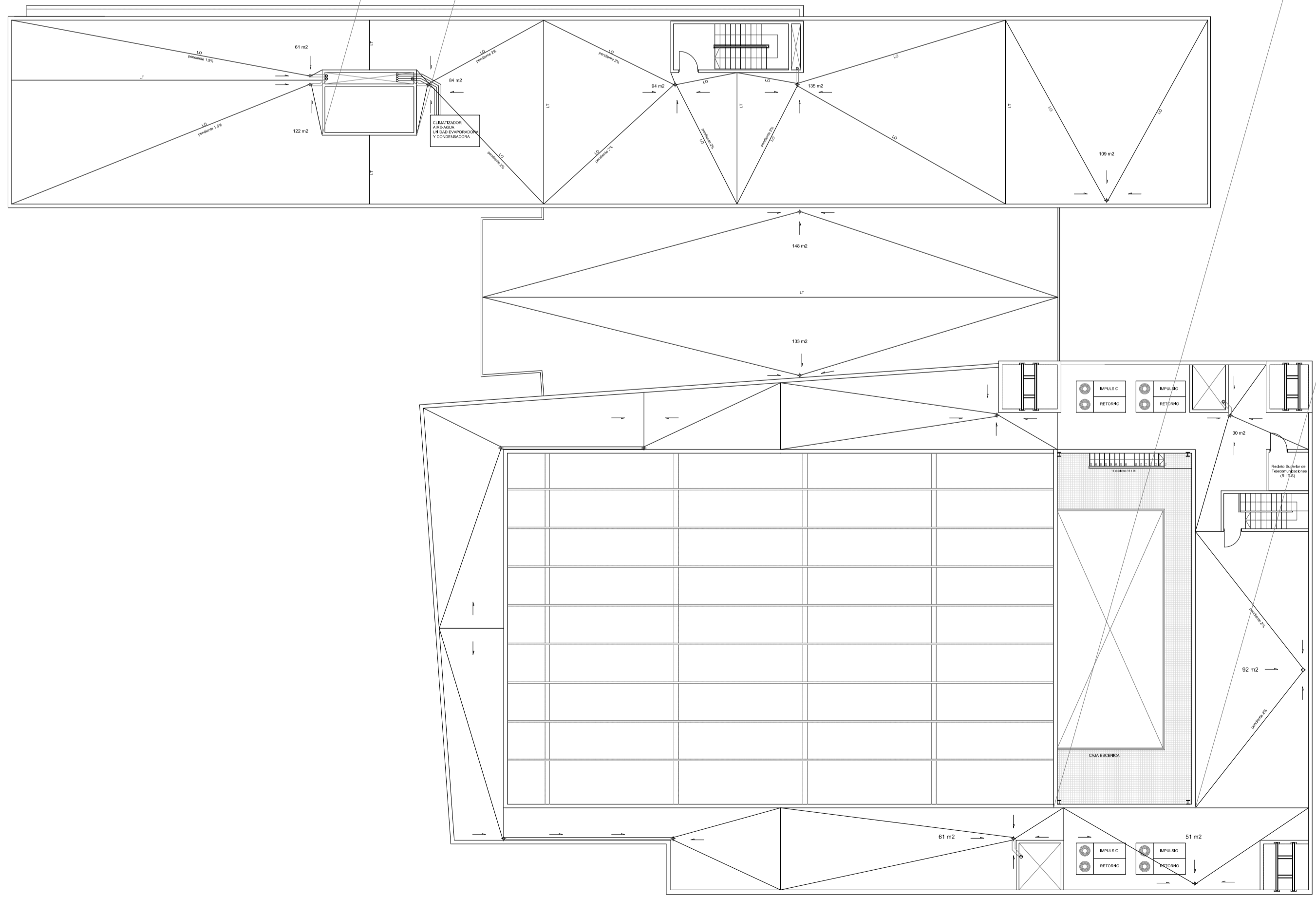
PLANTA CUBIERTA esc. 1/200
