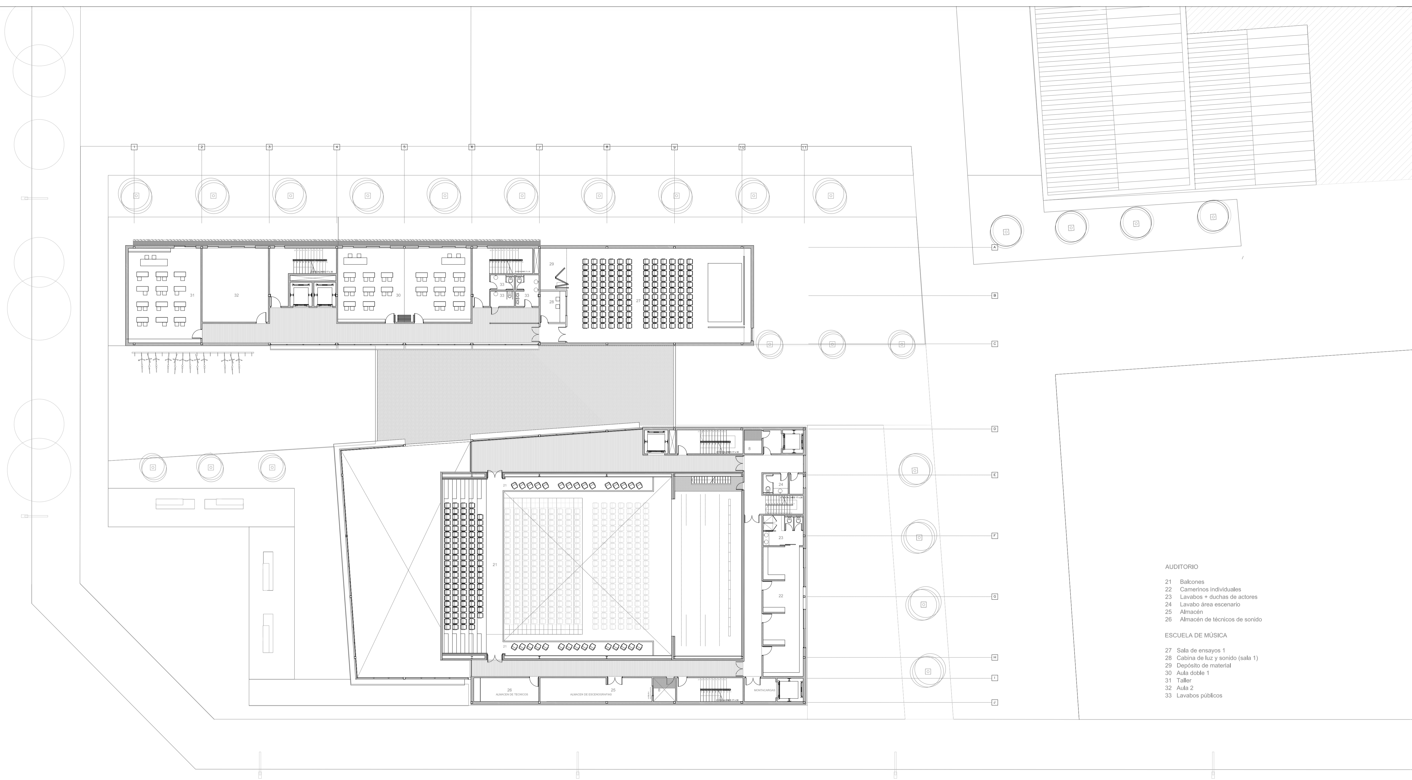
PLANTA 0 esc. 1/200
