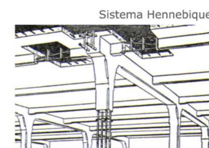
H=4,7m Estructura de formigó armat amb jàsseres acartellades Forjats de viguetes de formigó armat acartellades i revoltons creàtics
