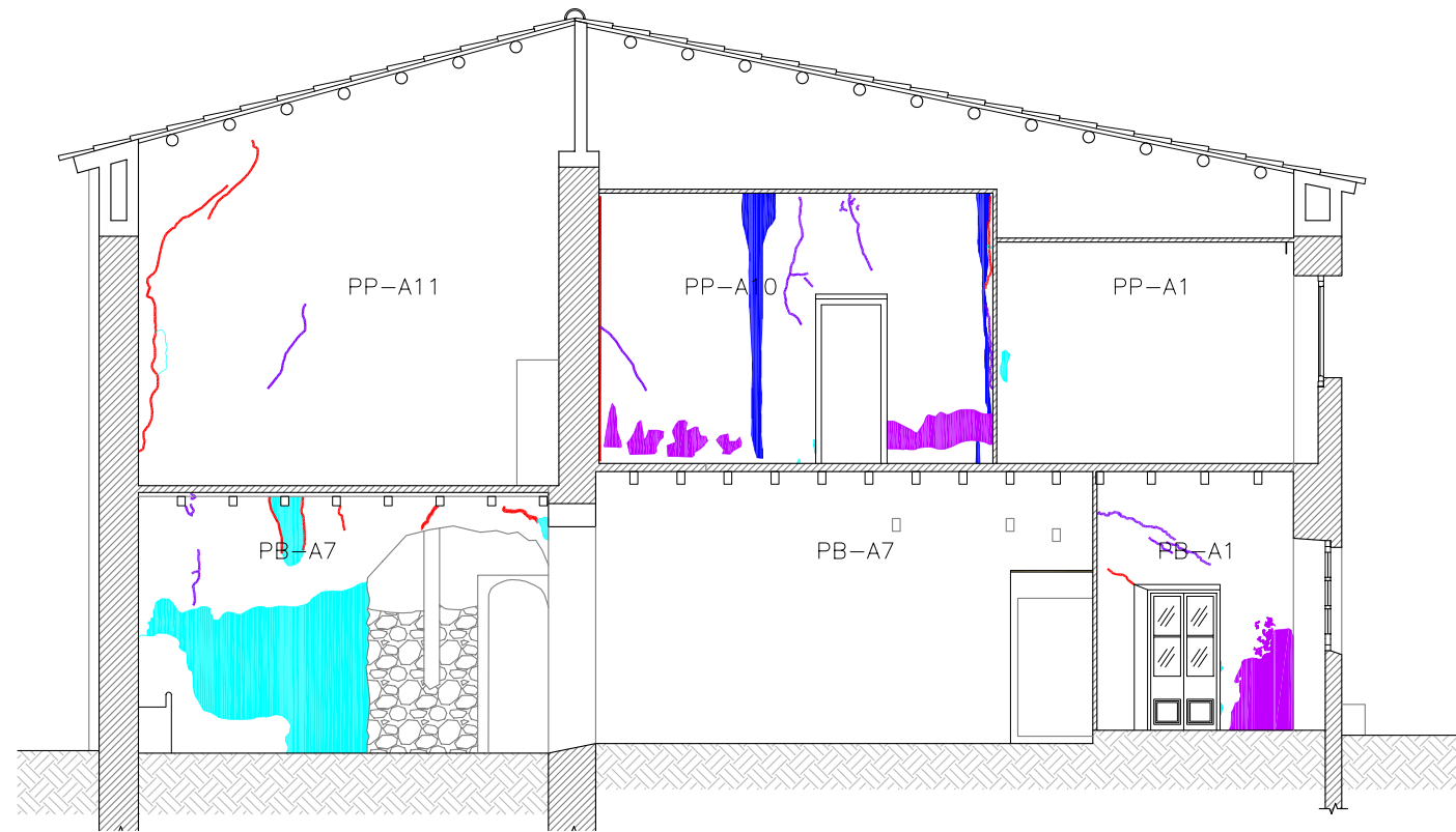
SECCIÓN E
