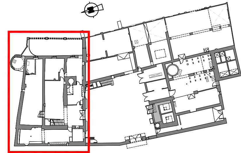
PLANTA BAJA E: 1/500
