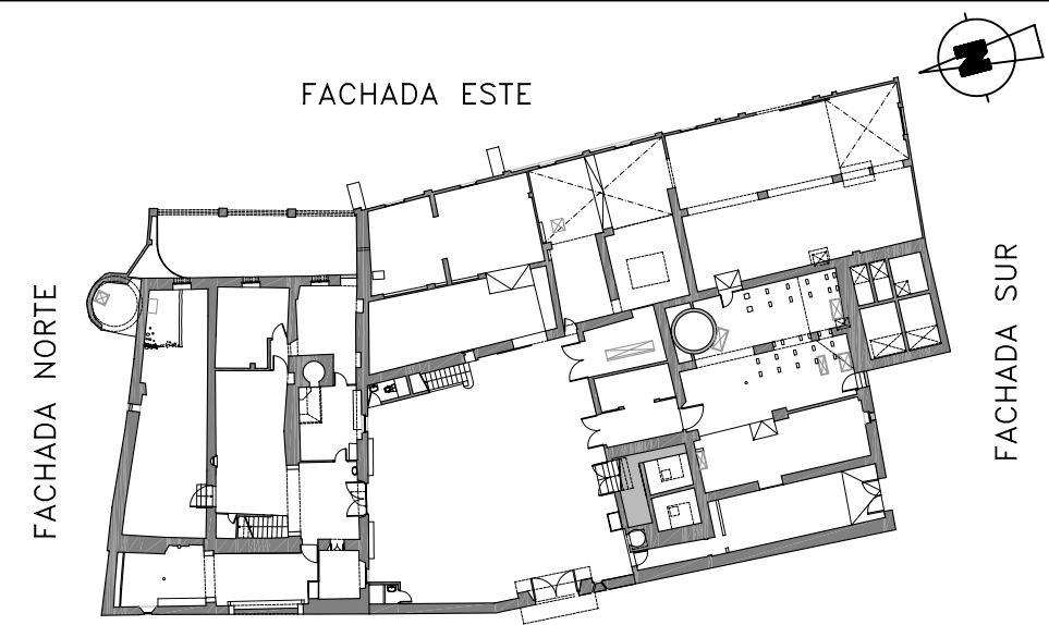
PLANTA BAJA E: 1/500
