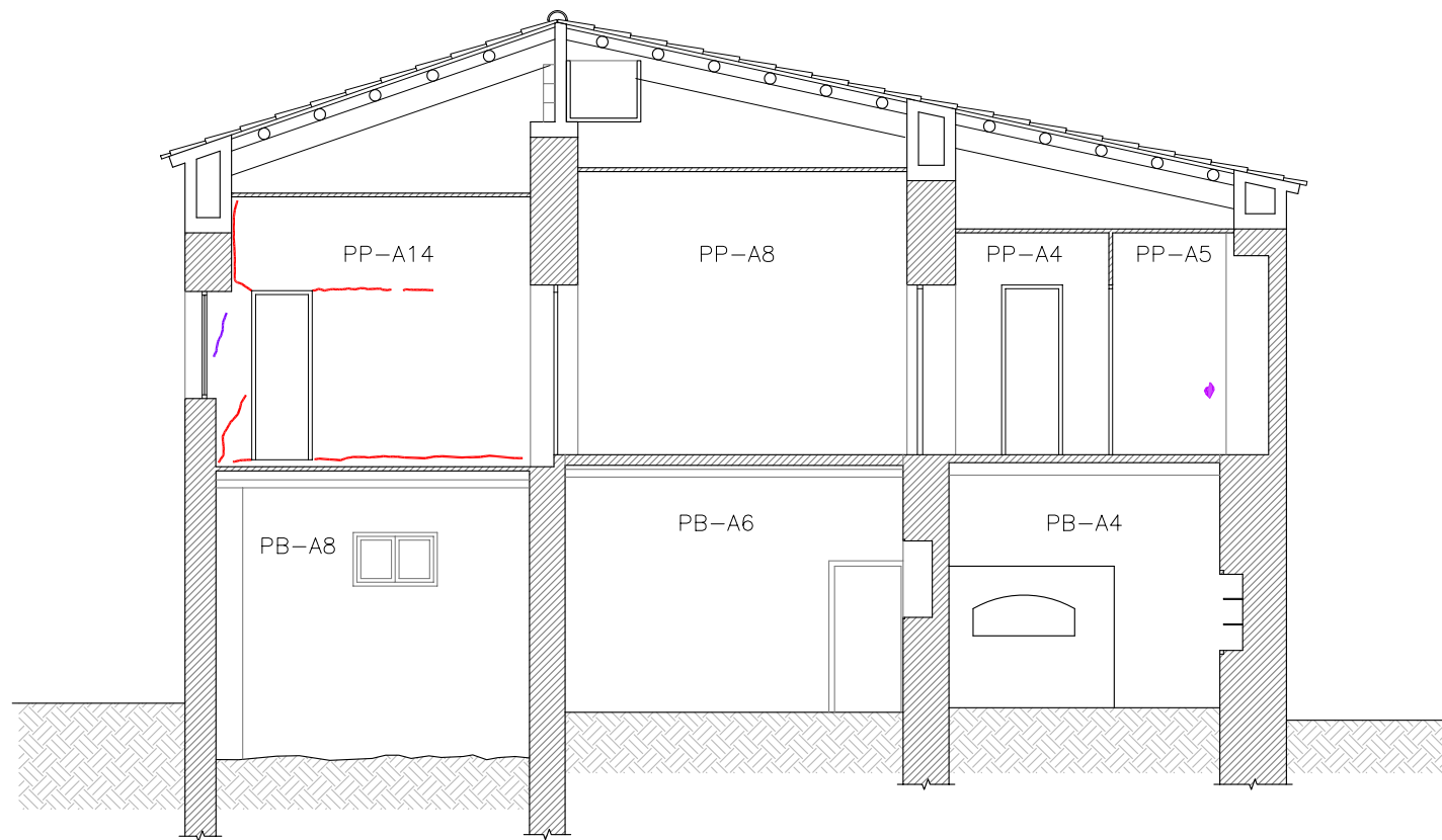
SECCIÓN H
