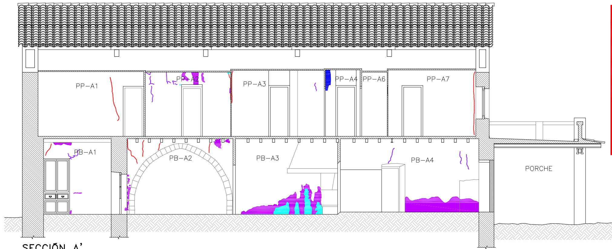
SECCIÓN A'
