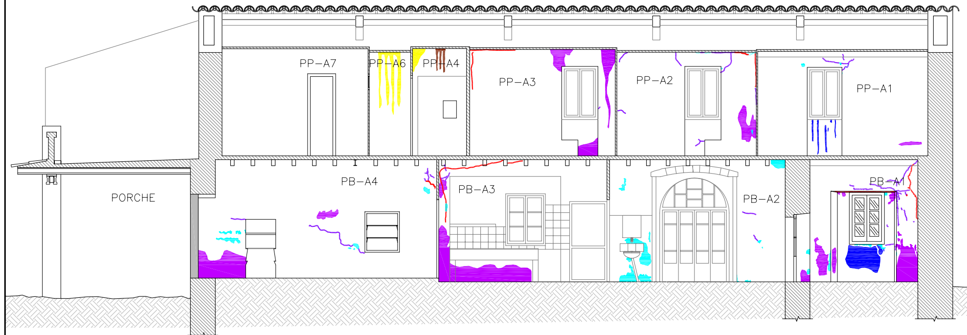
SECCIÓN A
