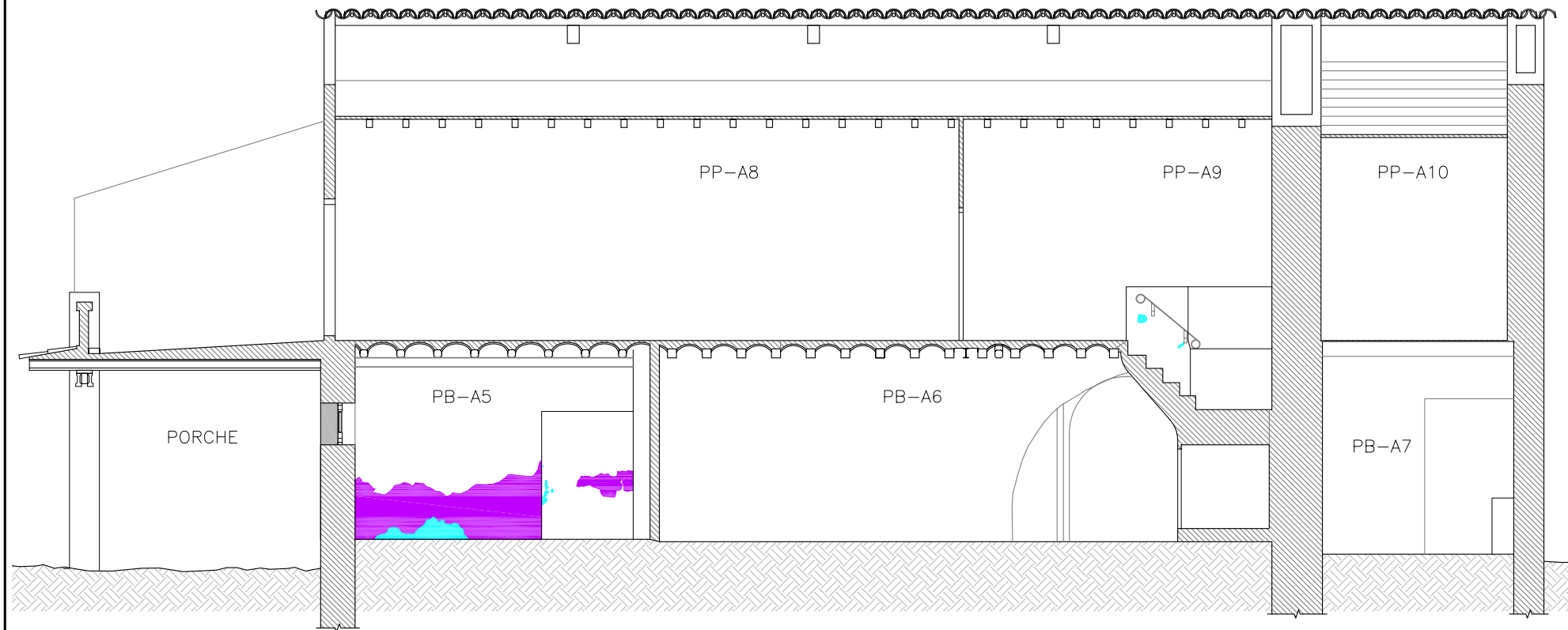
SECCIÓN C
