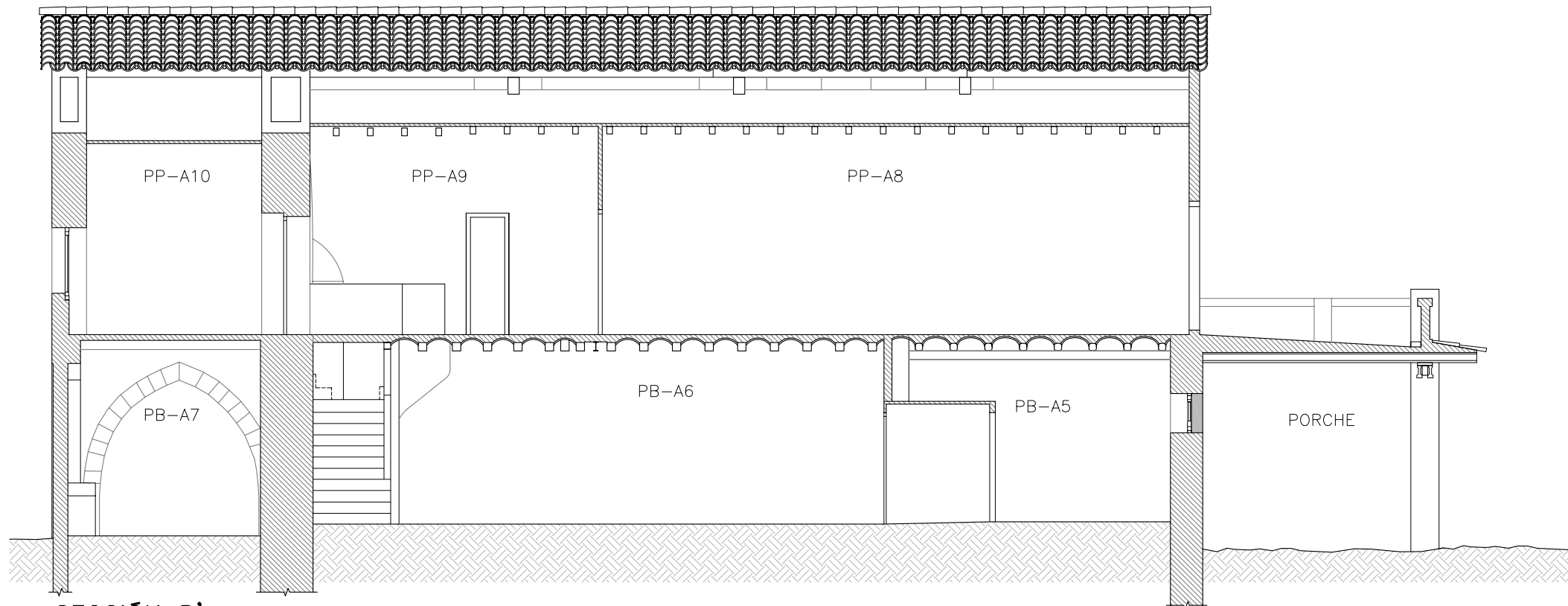
SECCIÓN B'
