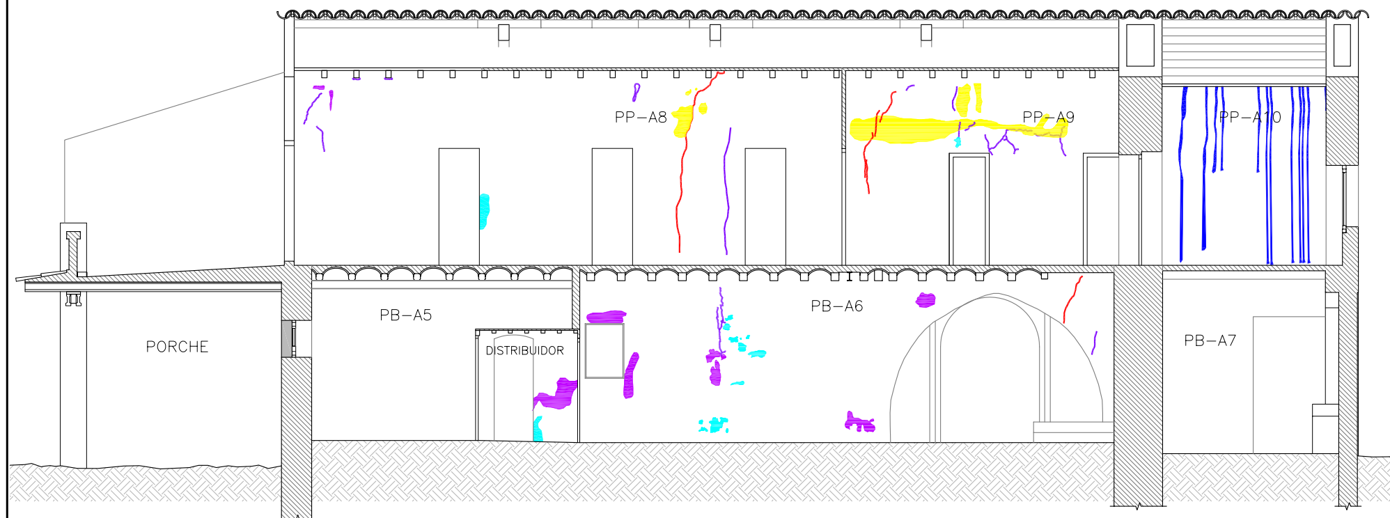
SECCIÓN B
