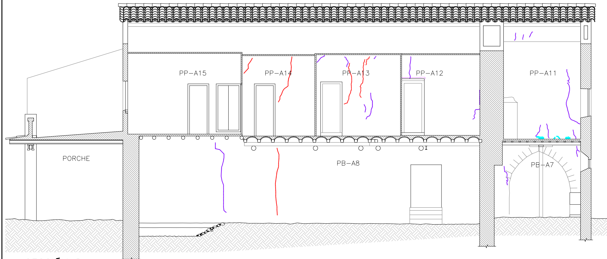
SECCIÓN D
