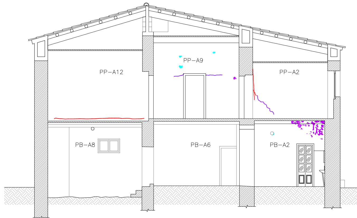
SECCIÓN F
